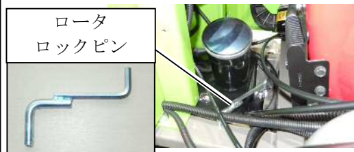
ロータロックピン収納位置
