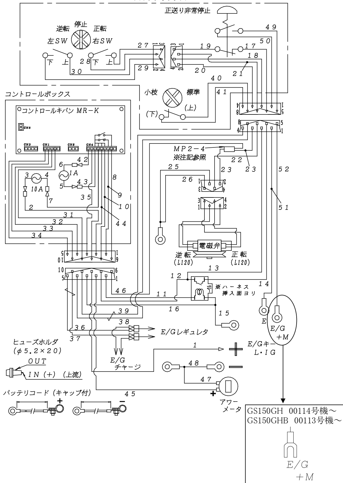
配線図 GS150GH スイッチボックス
