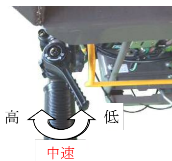
スロットルレバー
