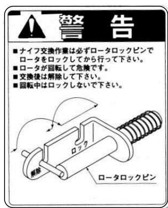
ロータロックピン
