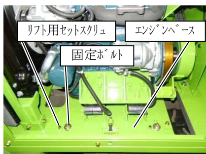
エンジンベース
