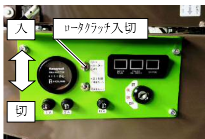
ロータクラッチスイッチ
