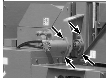
送りモータ・軸受取付部
