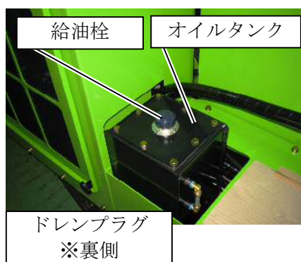
オイルタンク
