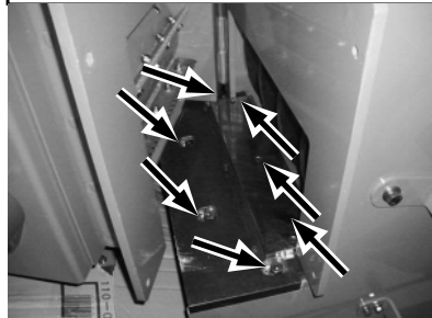
受刃取付ボルト・アジャスタボルト
