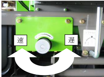
送り速度調整ダイヤル
