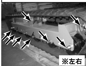
転輪・誘導輪固定ナット
