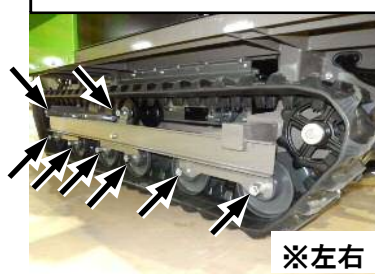
転輪・誘導輪固定ナット
