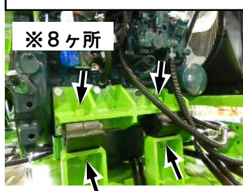
エンジン取付ナット
