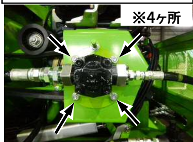
オイルポンプ固定ボルト・ナット
