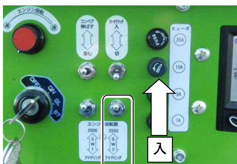
スロットルスイッチ2
