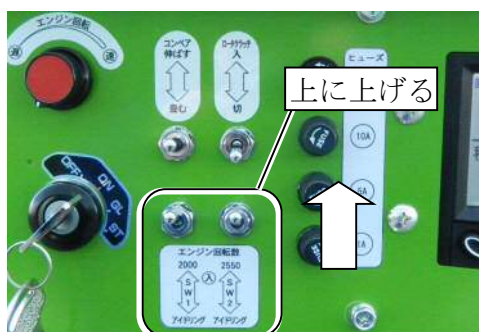
スロットルスイッチ
