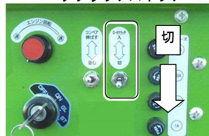
ロータクラッチスイッチ
