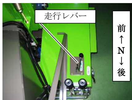
走行レバー
