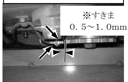
センサ固定ナット
