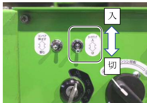
ロータクラッチスイッチ
