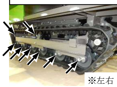
転輪・誘導輪固定ナット
