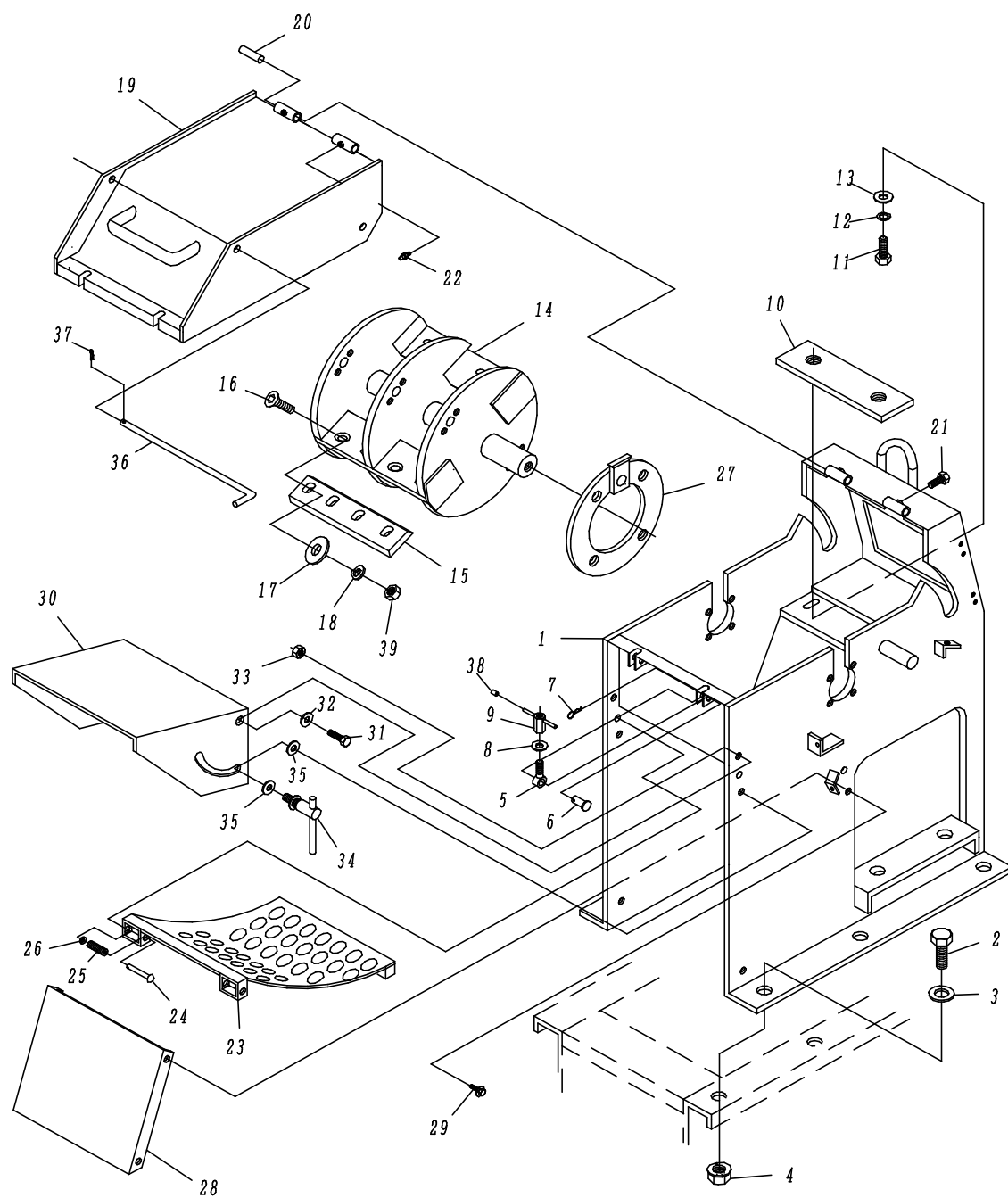
Fig. 6 ロータ系
