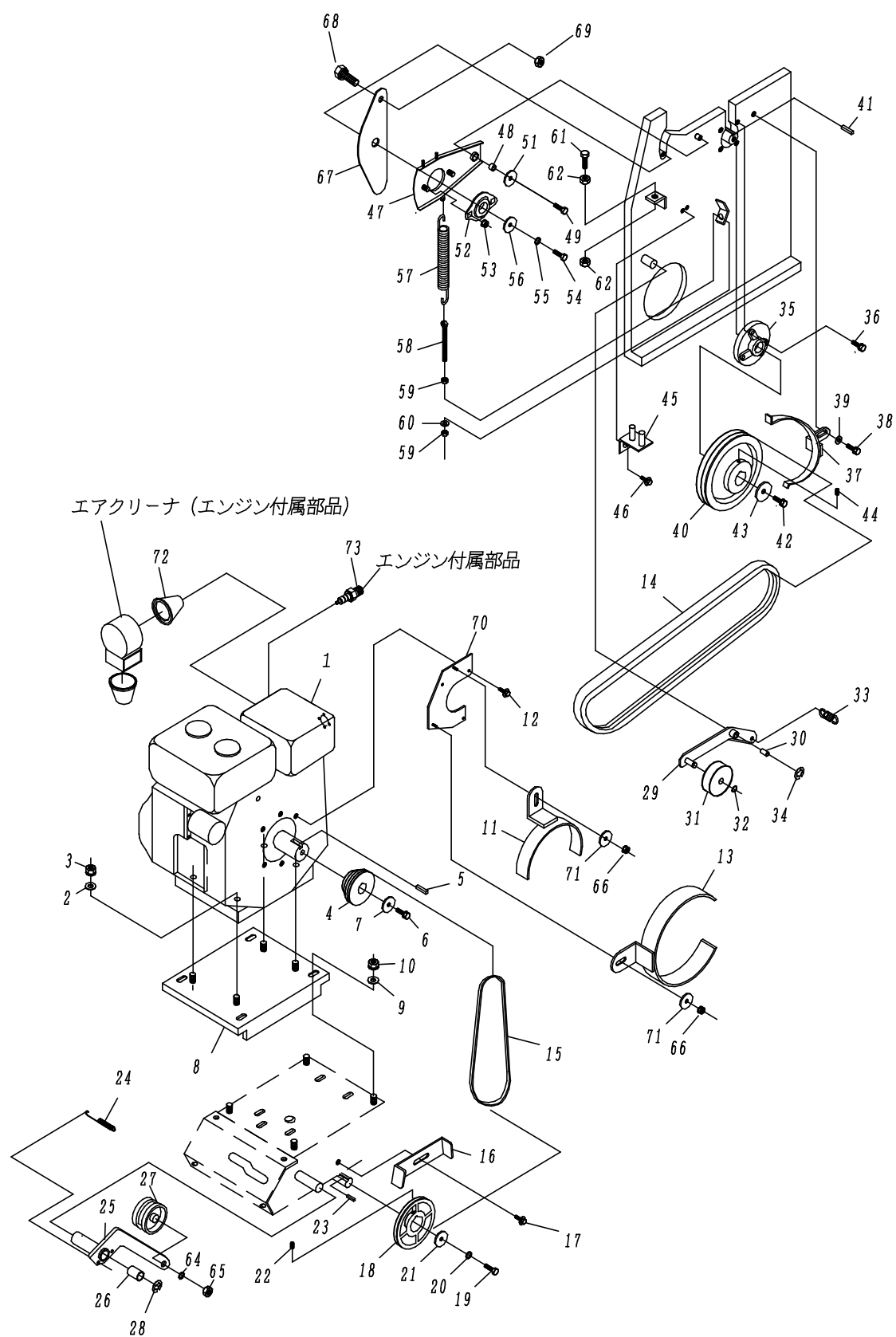
Fig. 4 エンジン系(2)
