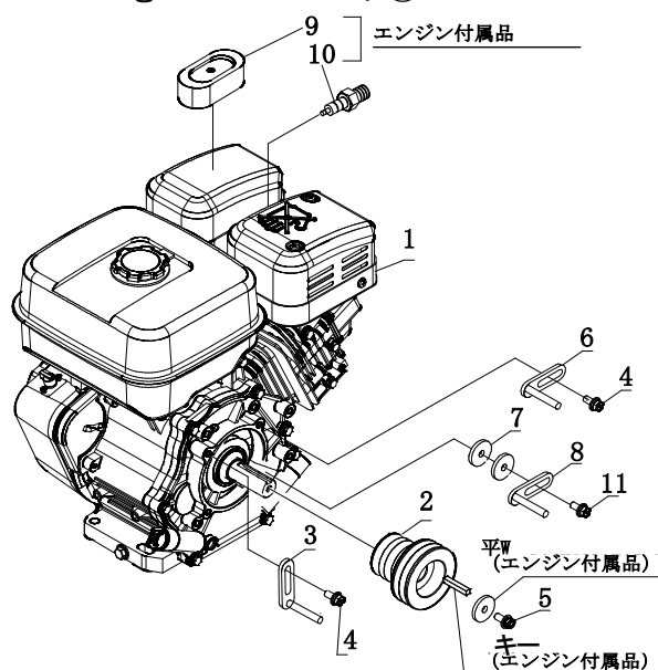
Fig. 6 エンジン系①
