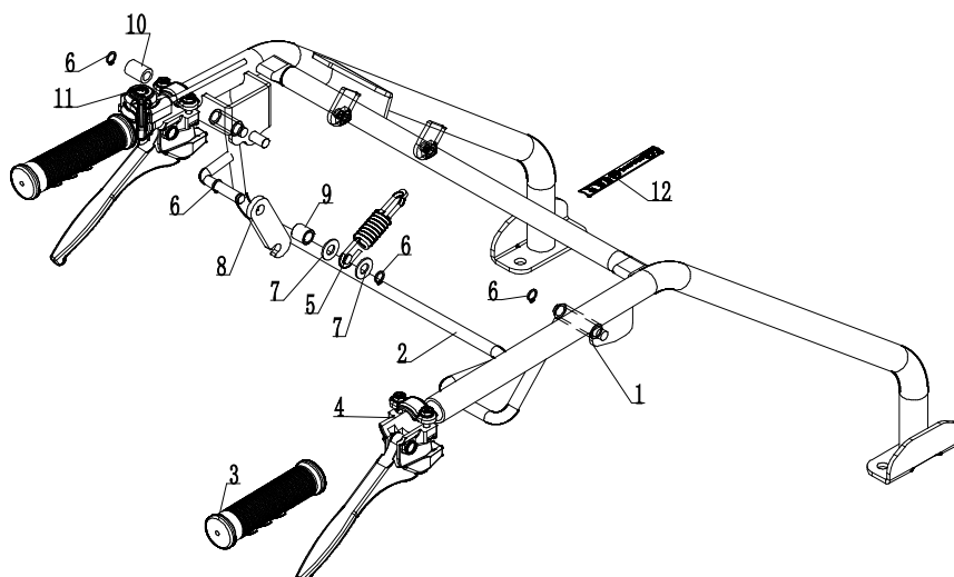
Fig. 4 ハンドル系①
