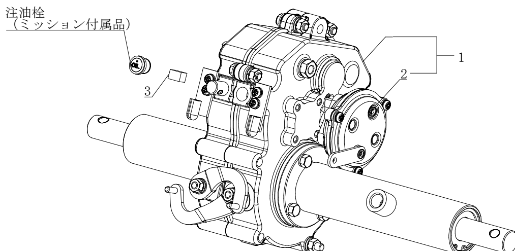
Fig. 5 ミッション系①
