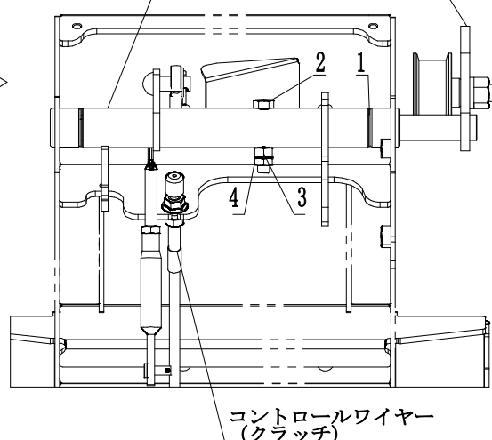
ブレーキリンク
