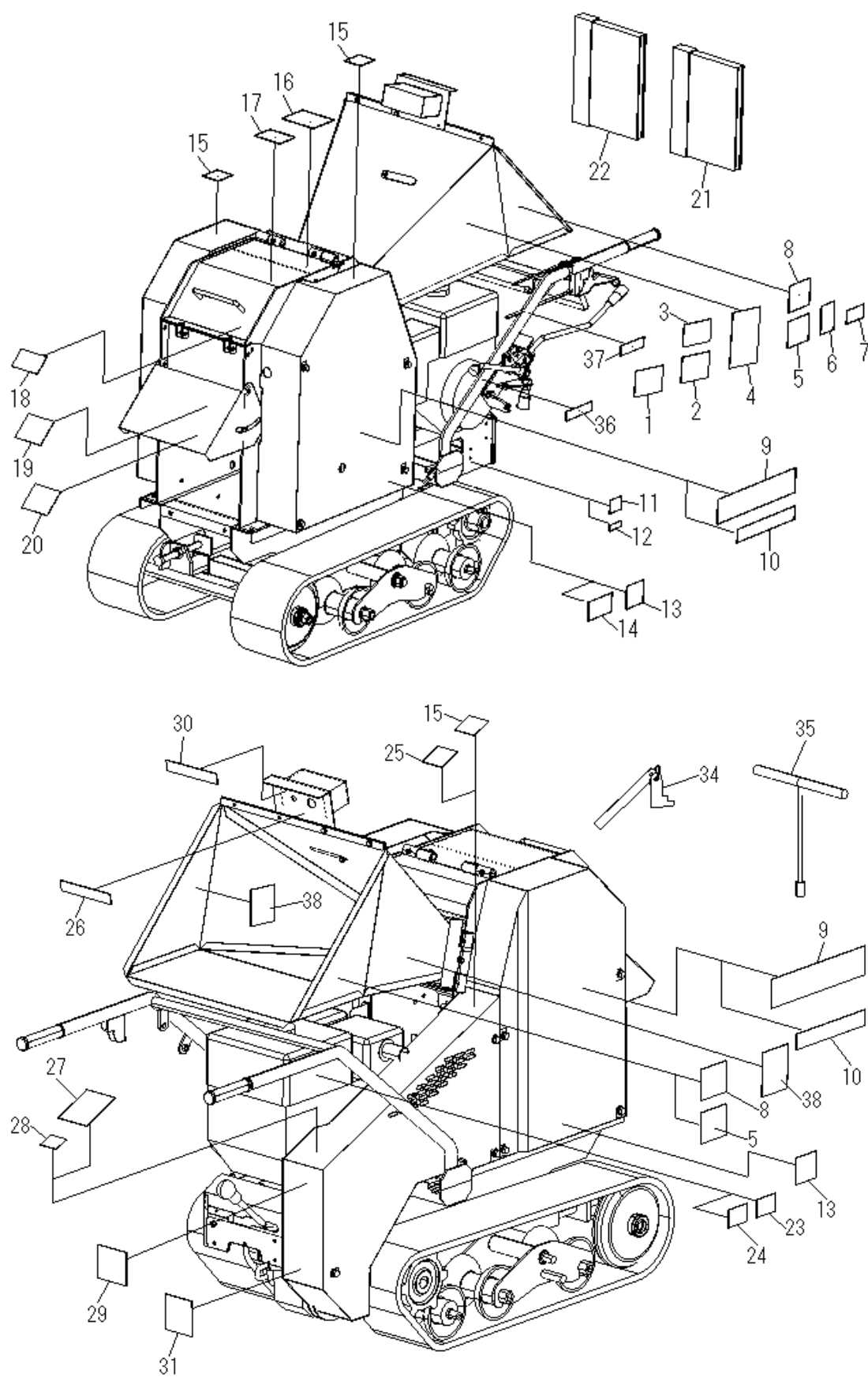
Fig. 15 ステッカー系
