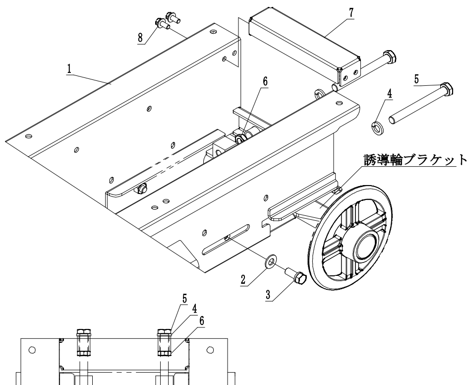
Fig. 1 フレーム系
