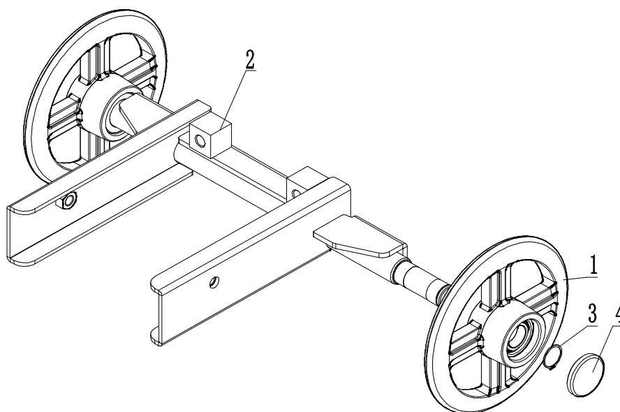
Fig. 3 遊導輪系
