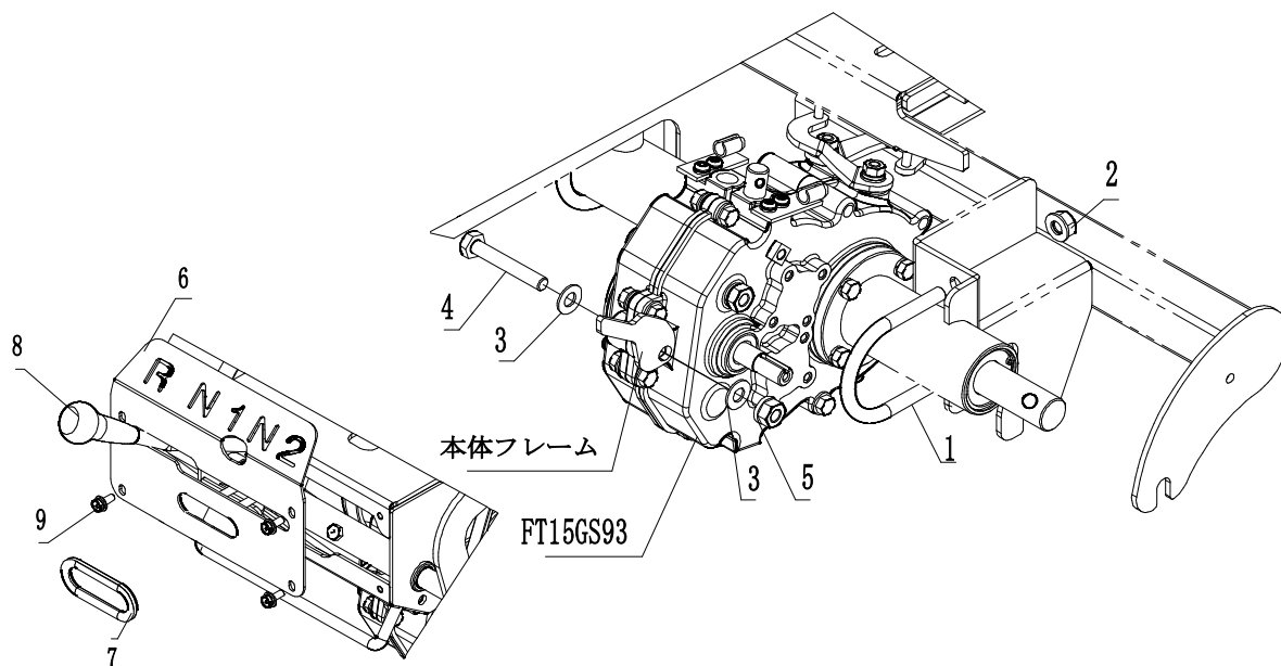
Fig. 5 ミッション系②
