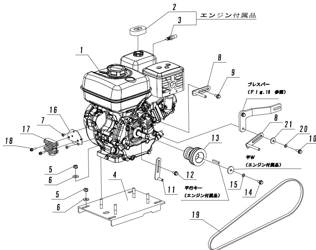
Fig. 9 エンジン
