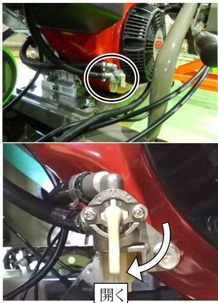
燃料コック
