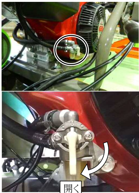
燃料コック
