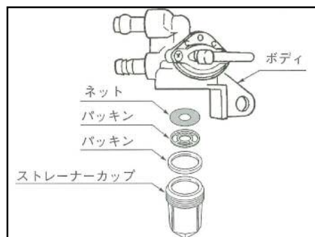
燃料コック
