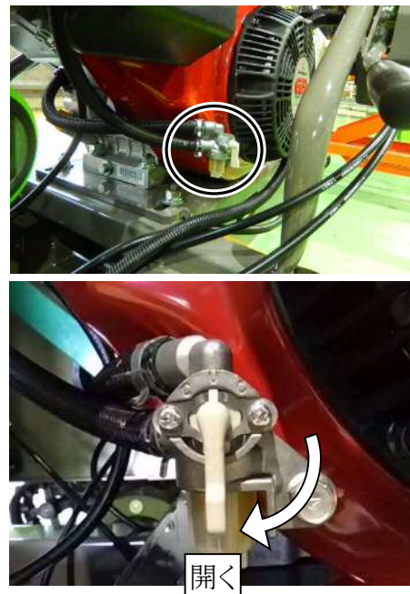
燃料コック
