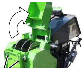
固定ネジ
