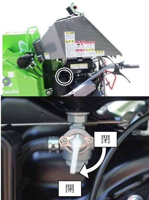
燃料コック
