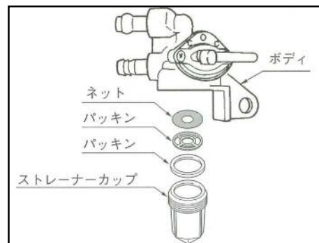
燃料コック
