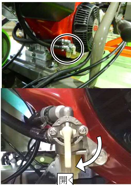
燃料コック
