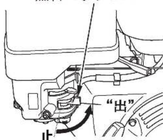
燃料コックレバー
