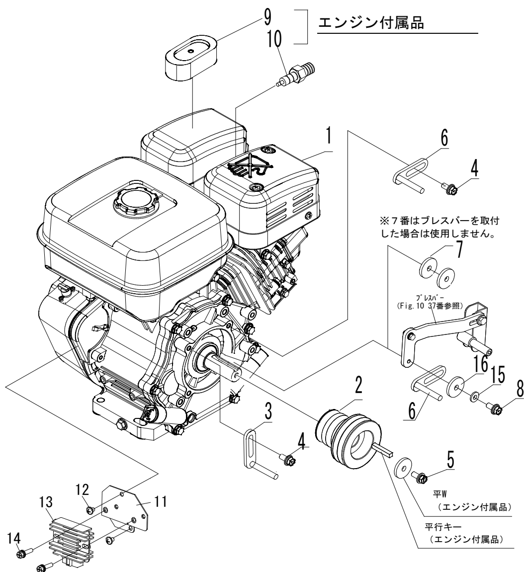
Fig. 6 エンジン系①
