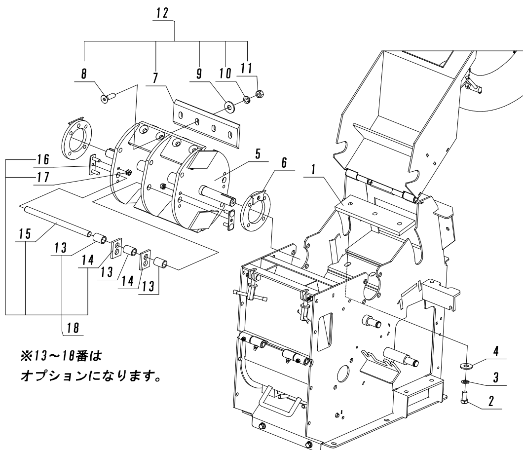
Fig. 13 ロータジク
