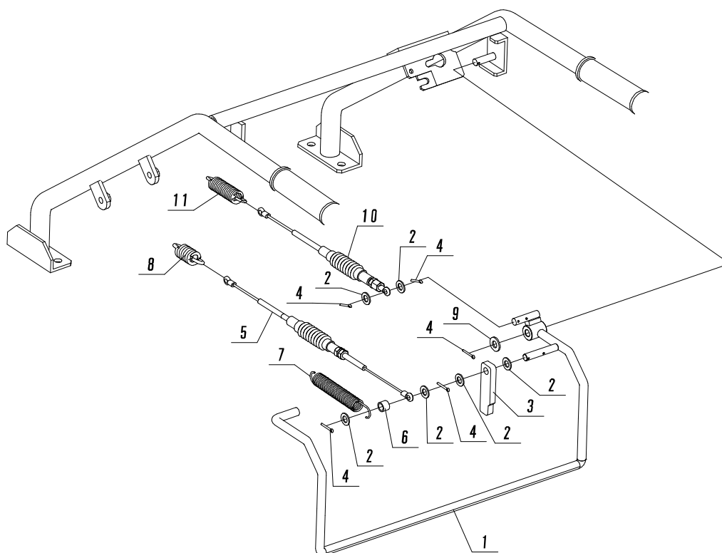
Fig. 6 走行レバー
