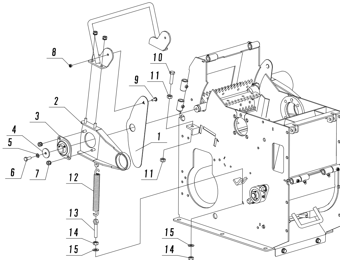
Fig. 23 フィーダR
