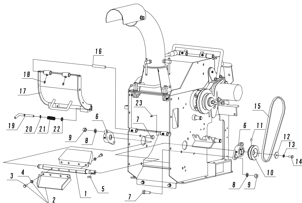
Fig. 18 ブロワ
