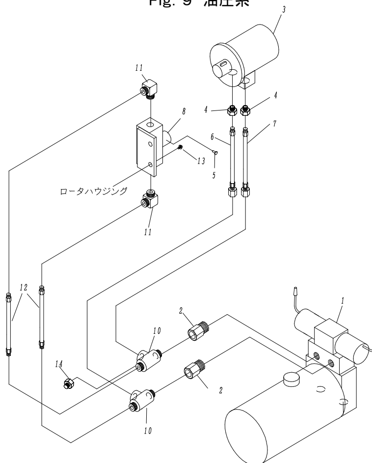
Fig. 9 油圧系
