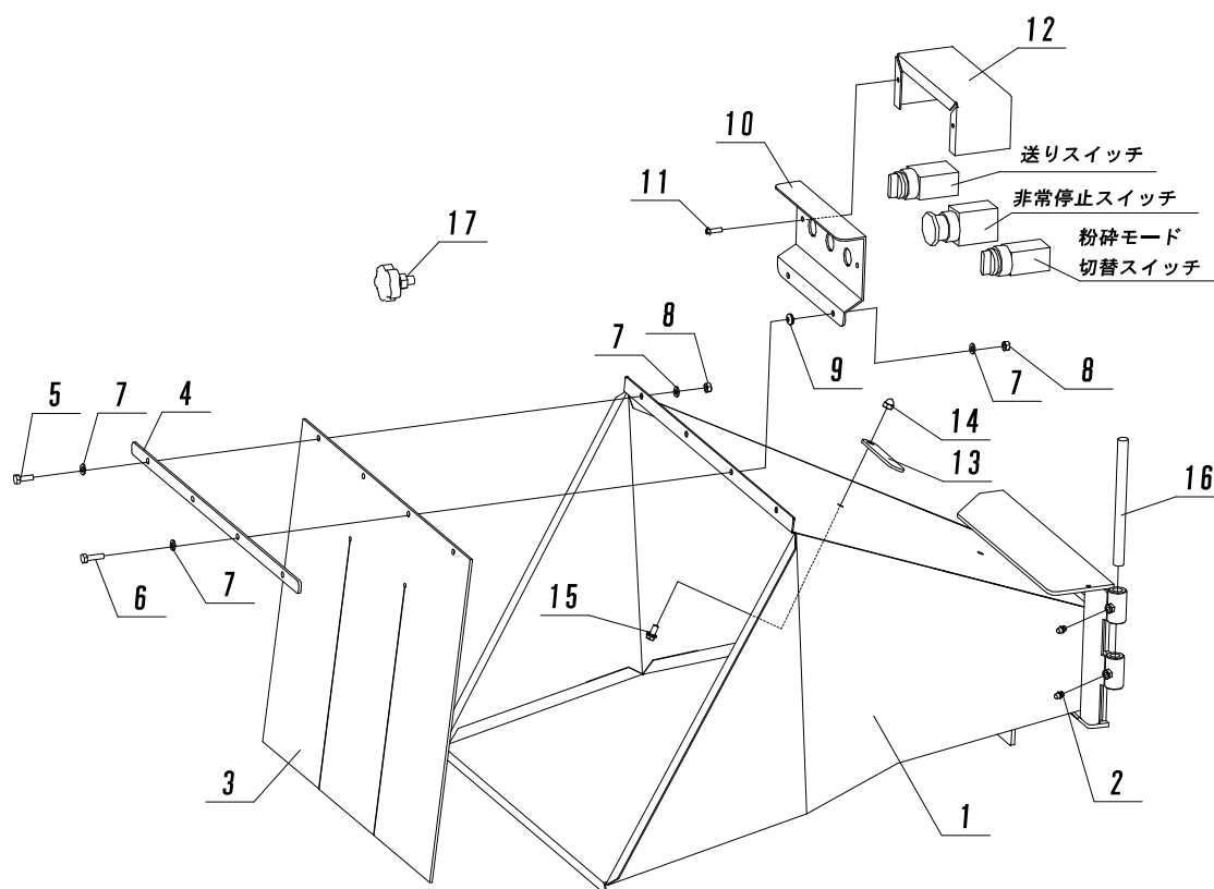
Fig. 24 ホツパ
