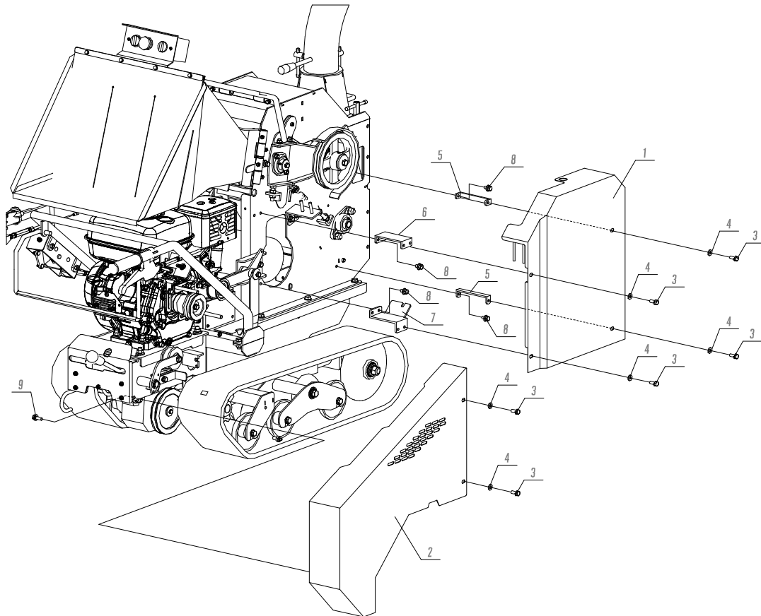
Fig. 25 カバー-R
