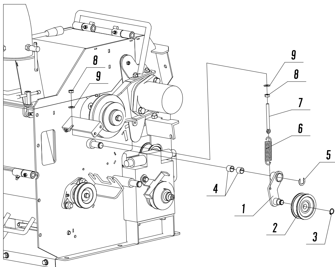
Fig. 19 Bテンションアーム
