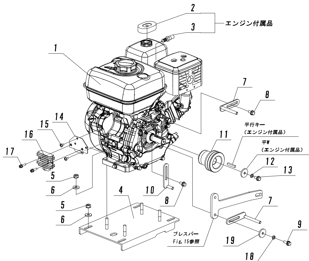
Fig. 11 エンジン
