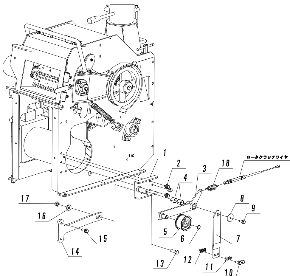
Fig. 15 Rテンションアーム、ブレスバー
