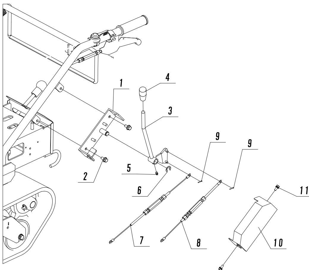
Fig. 7 Rレバー
