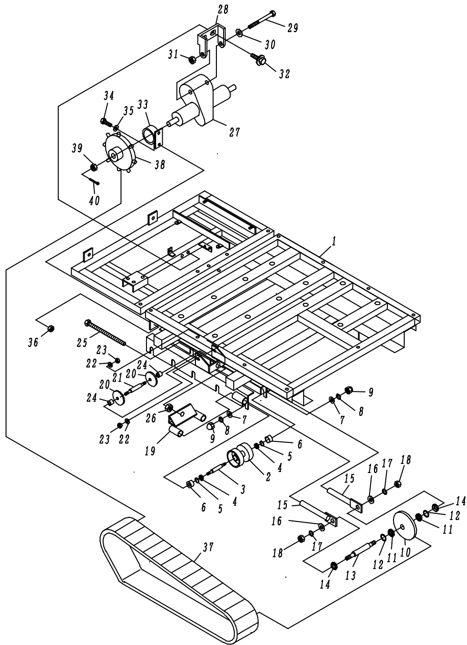
Fig. 1-1 フレーム系
