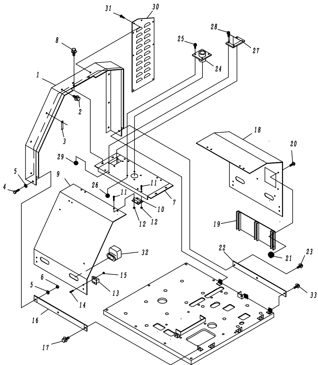
Fig. 9-1 カバー系
