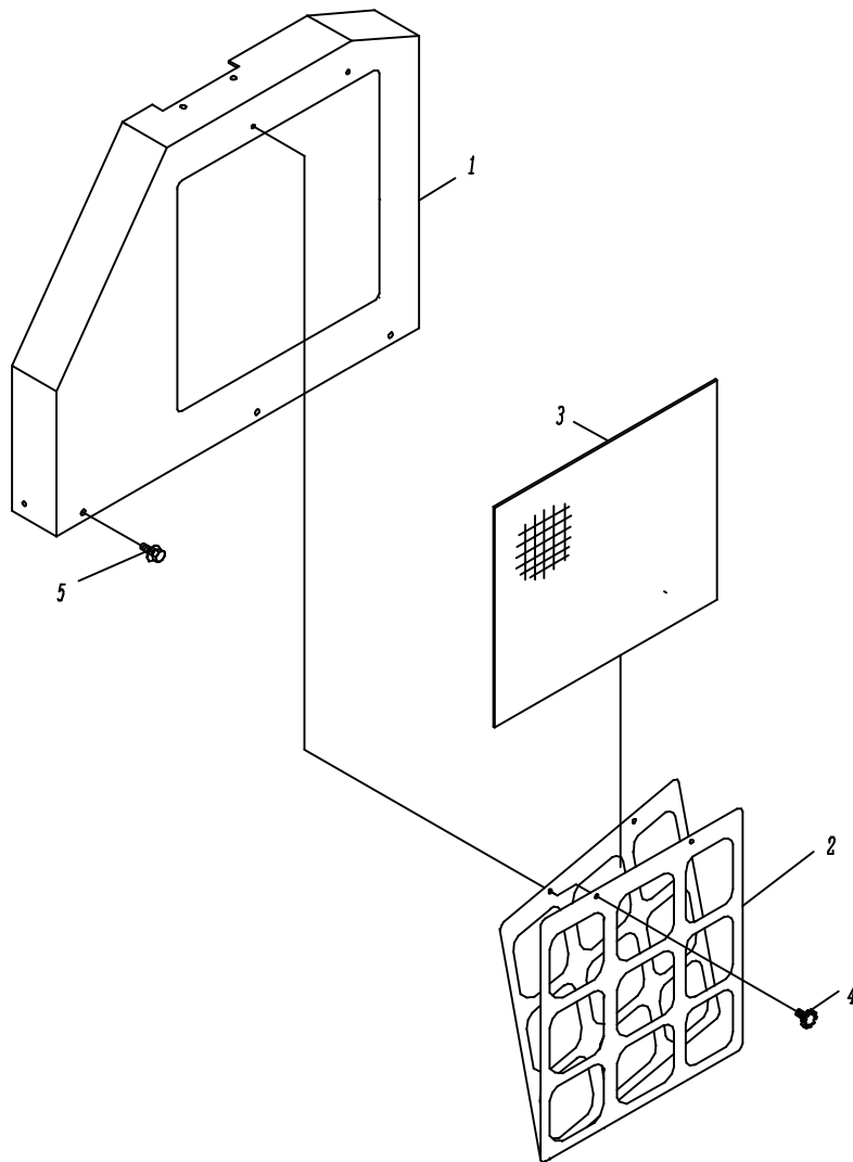
Fig. 9-2 カバー系
