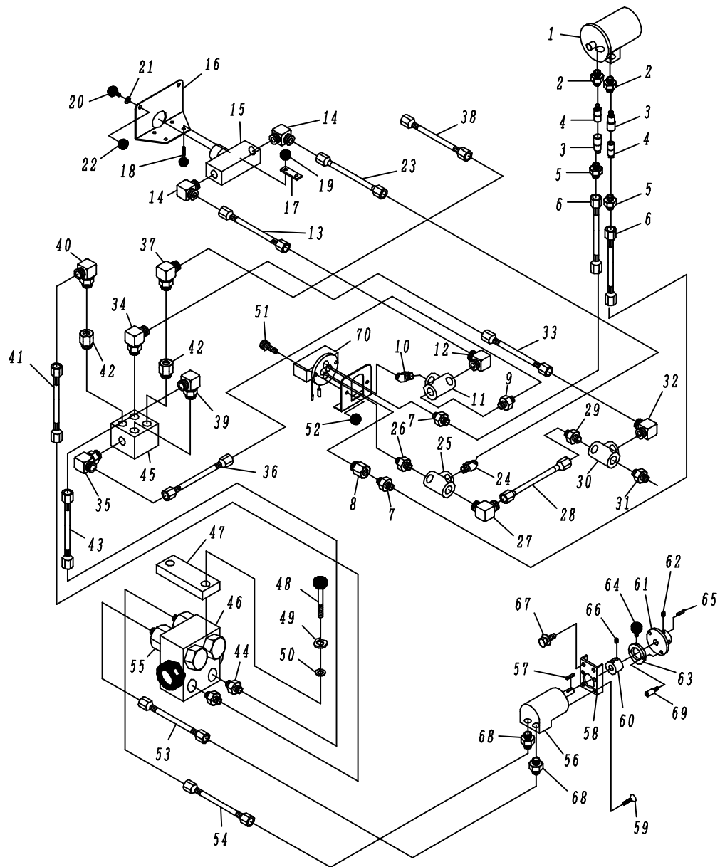
Fig. 3-1 油压系 (1)
