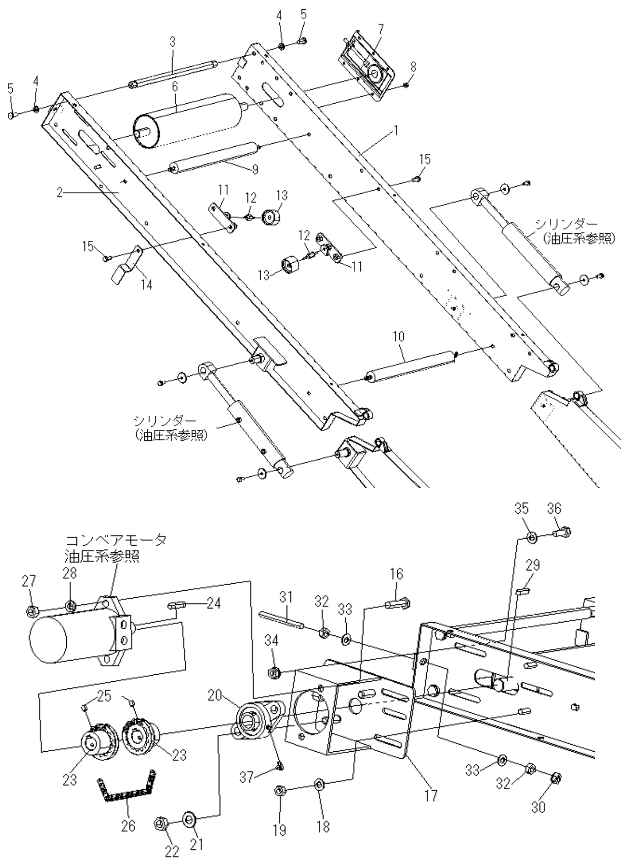
Fig. 23-2 排出コンベア
