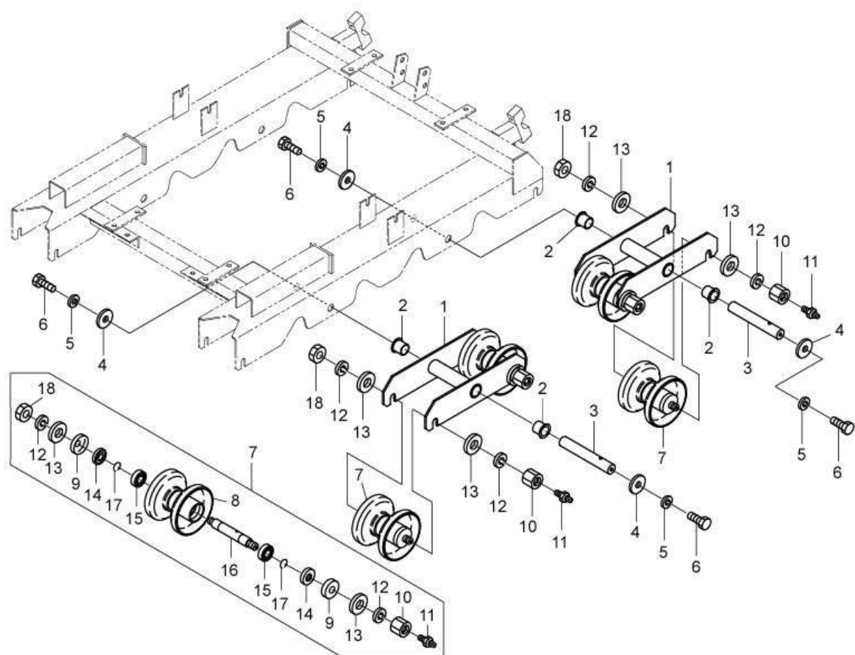
Fig. 7 轉輪系(2)
