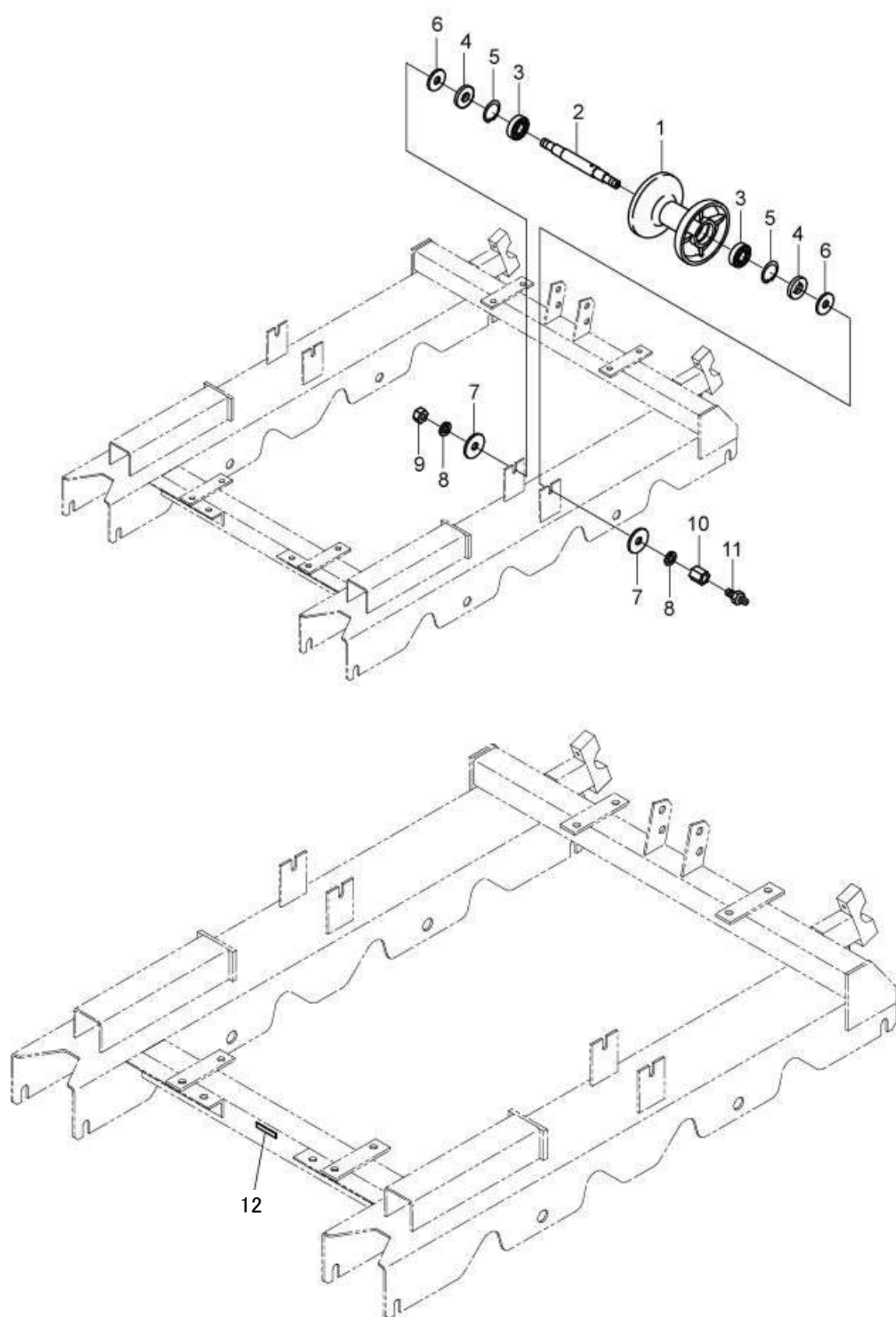
Fig. 8 転輪系(3)
