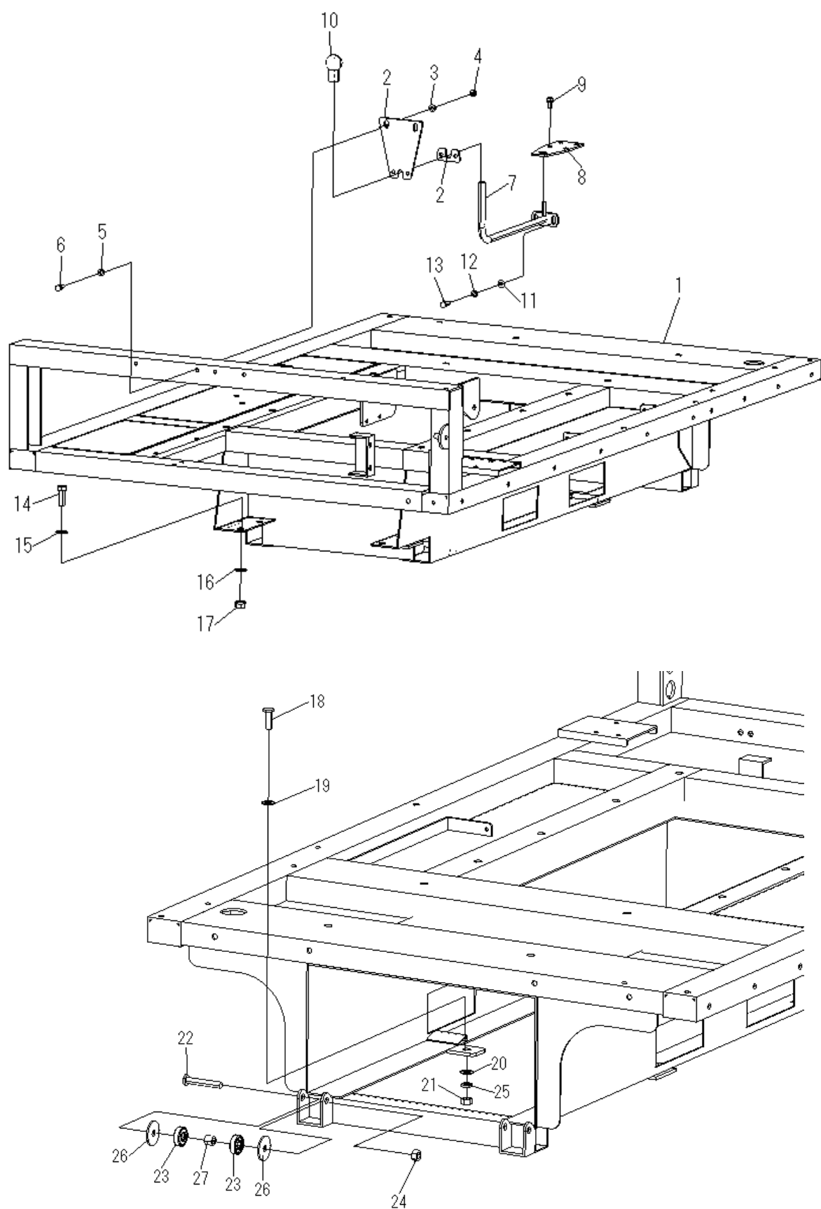
Fig. 10 フレーム系
