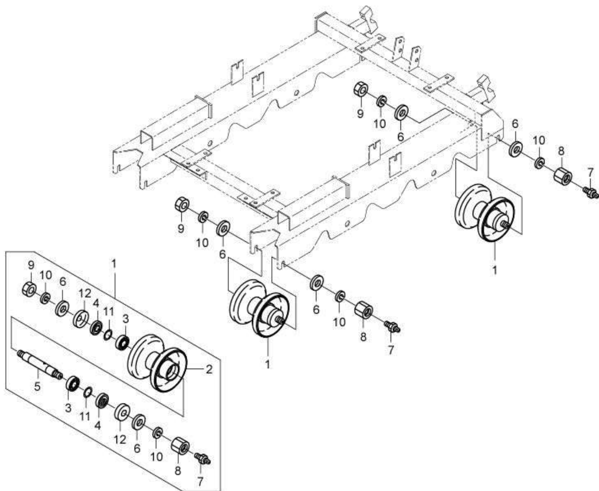
Fig. 6 転輪系(1)
