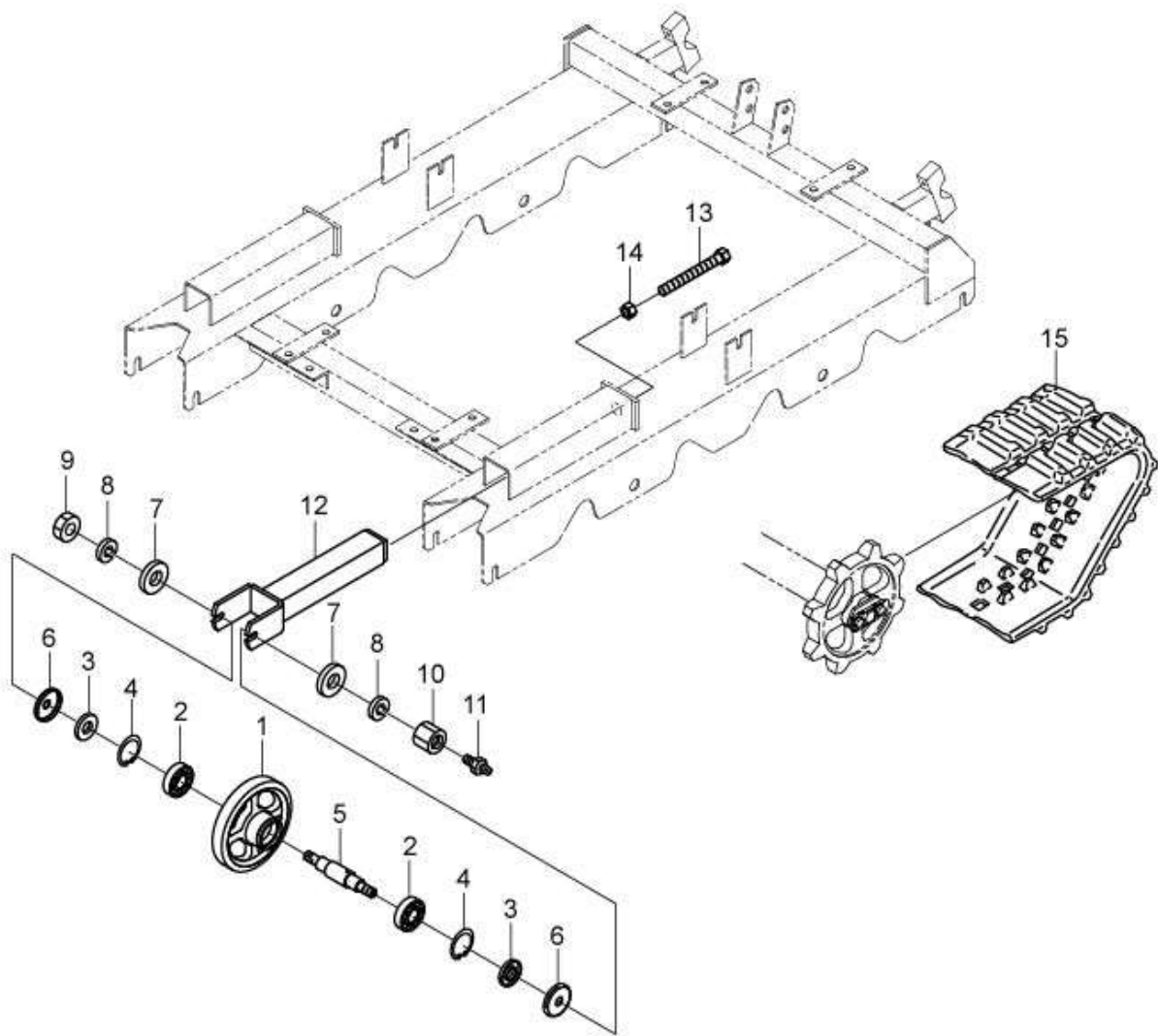
Fig. 9 クローラ系
