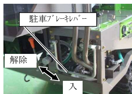
駐車ブレーキレバー
