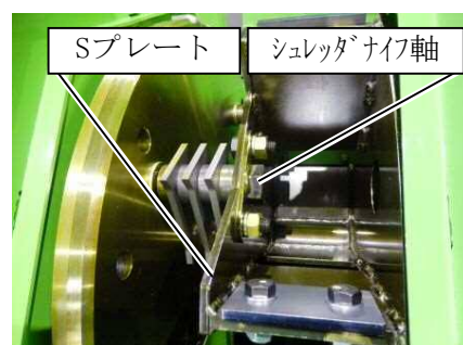
シュレッダナイフ
