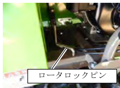
ロータロックピンの収納位置
