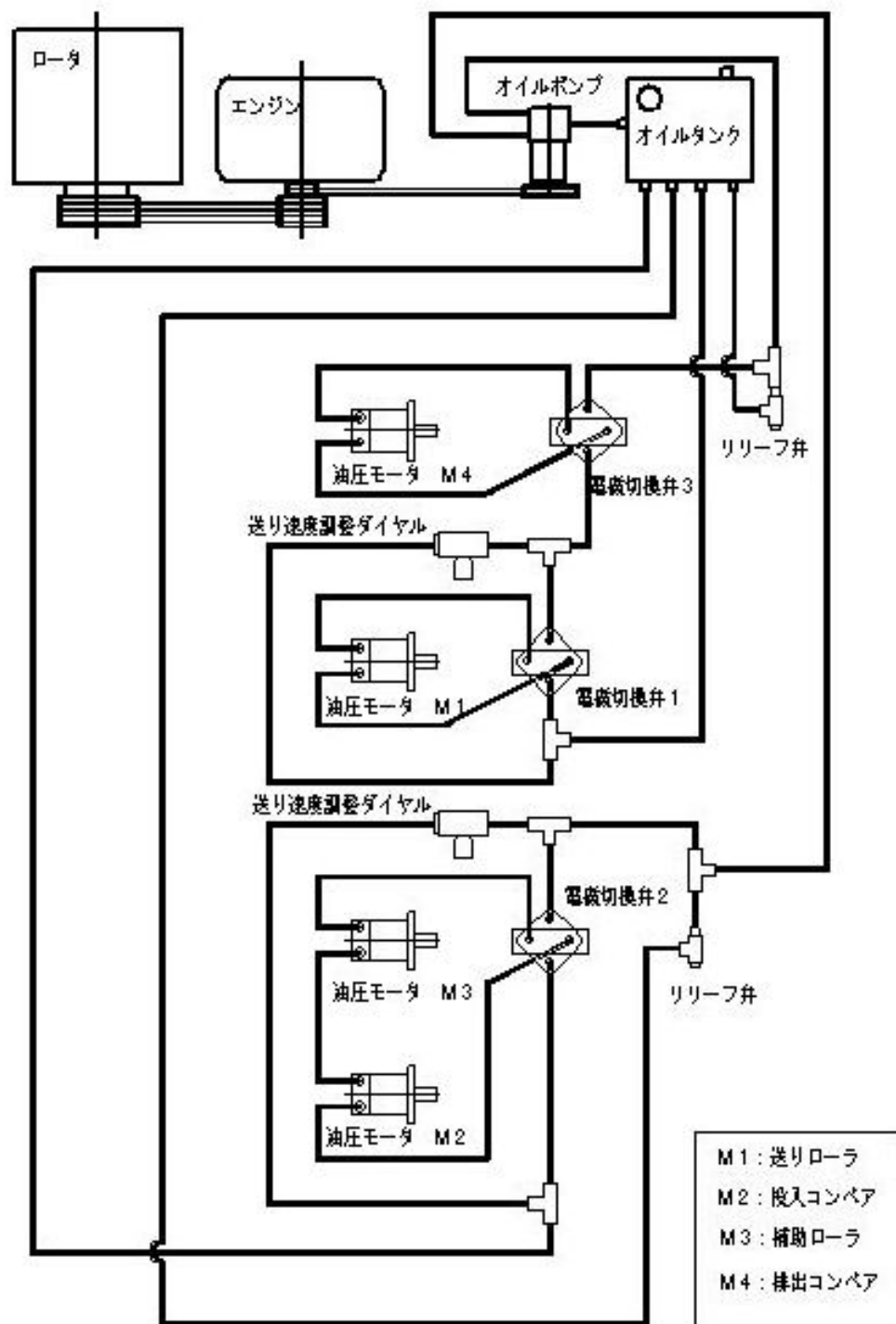
油圧配管図
