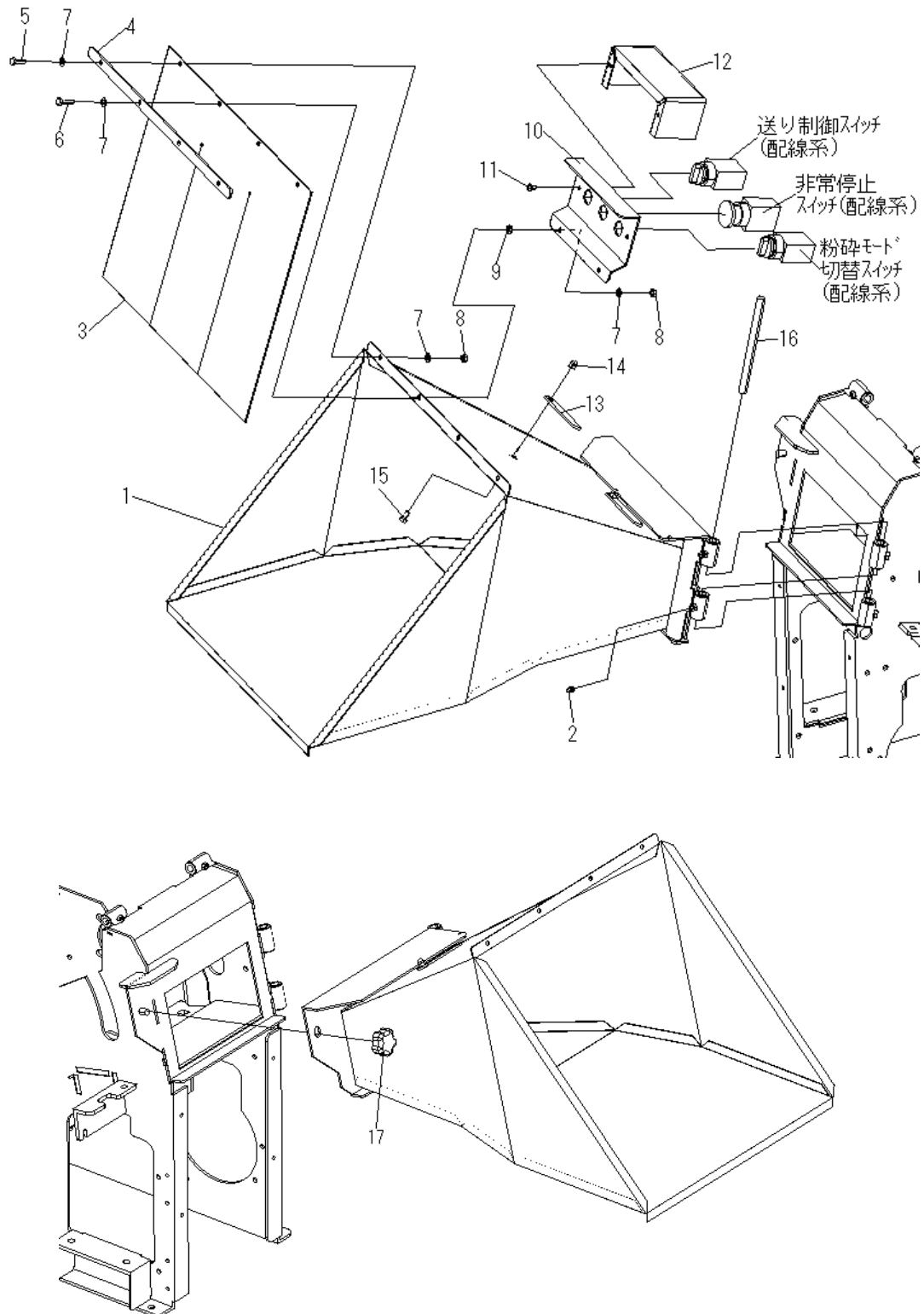
Fig. 14 ホツパ系
