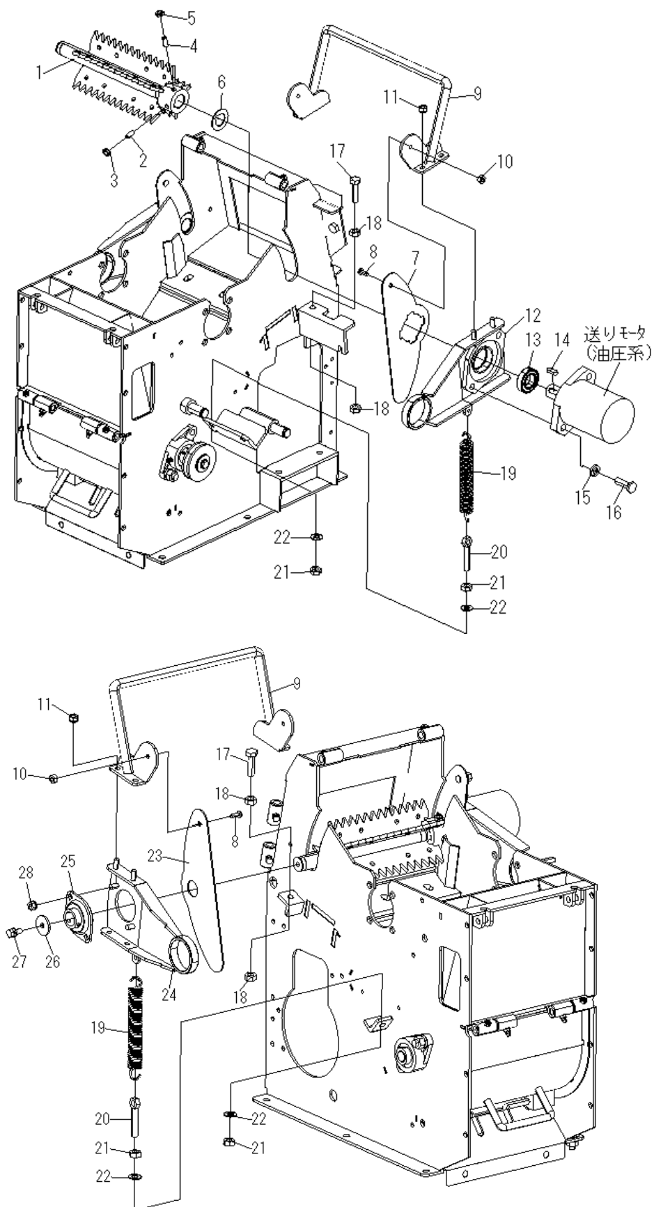
Fig. 13 フィーダ系
