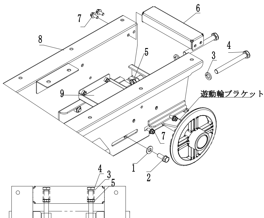
Fig. 1 フレーム系
