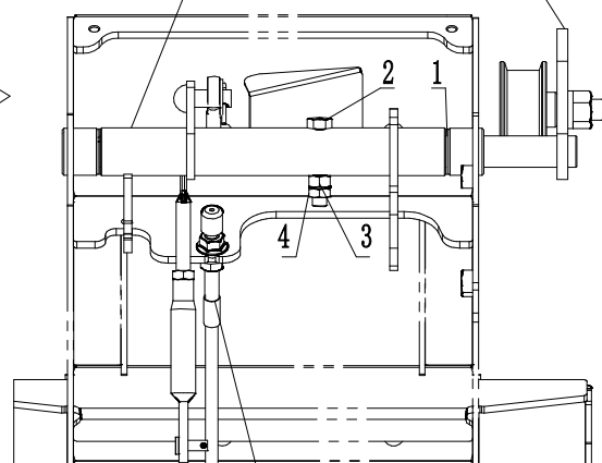
コントロールワイヤー (クラッチ)
