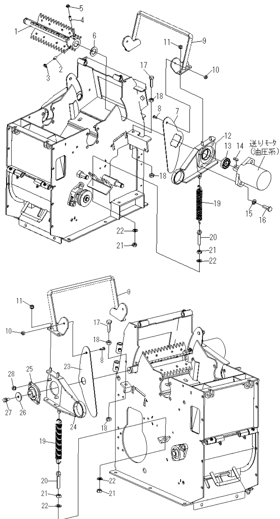
Fig. 13 フィーダ系
