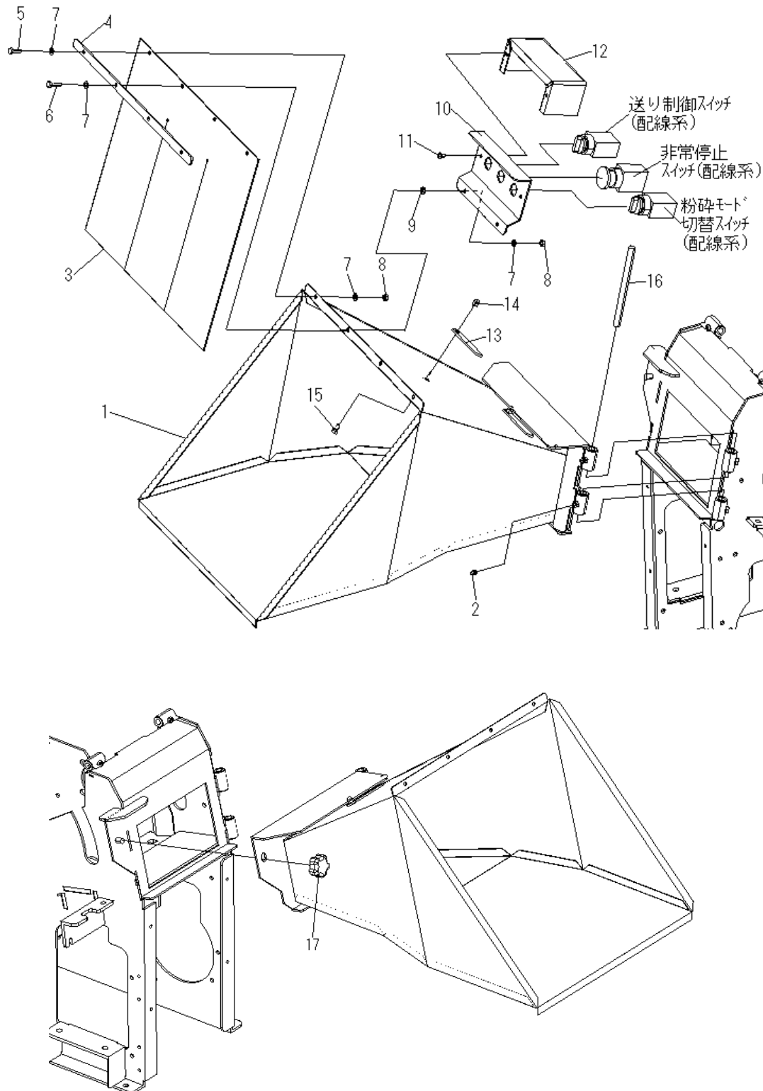
Fig. 14 ホツパ系
