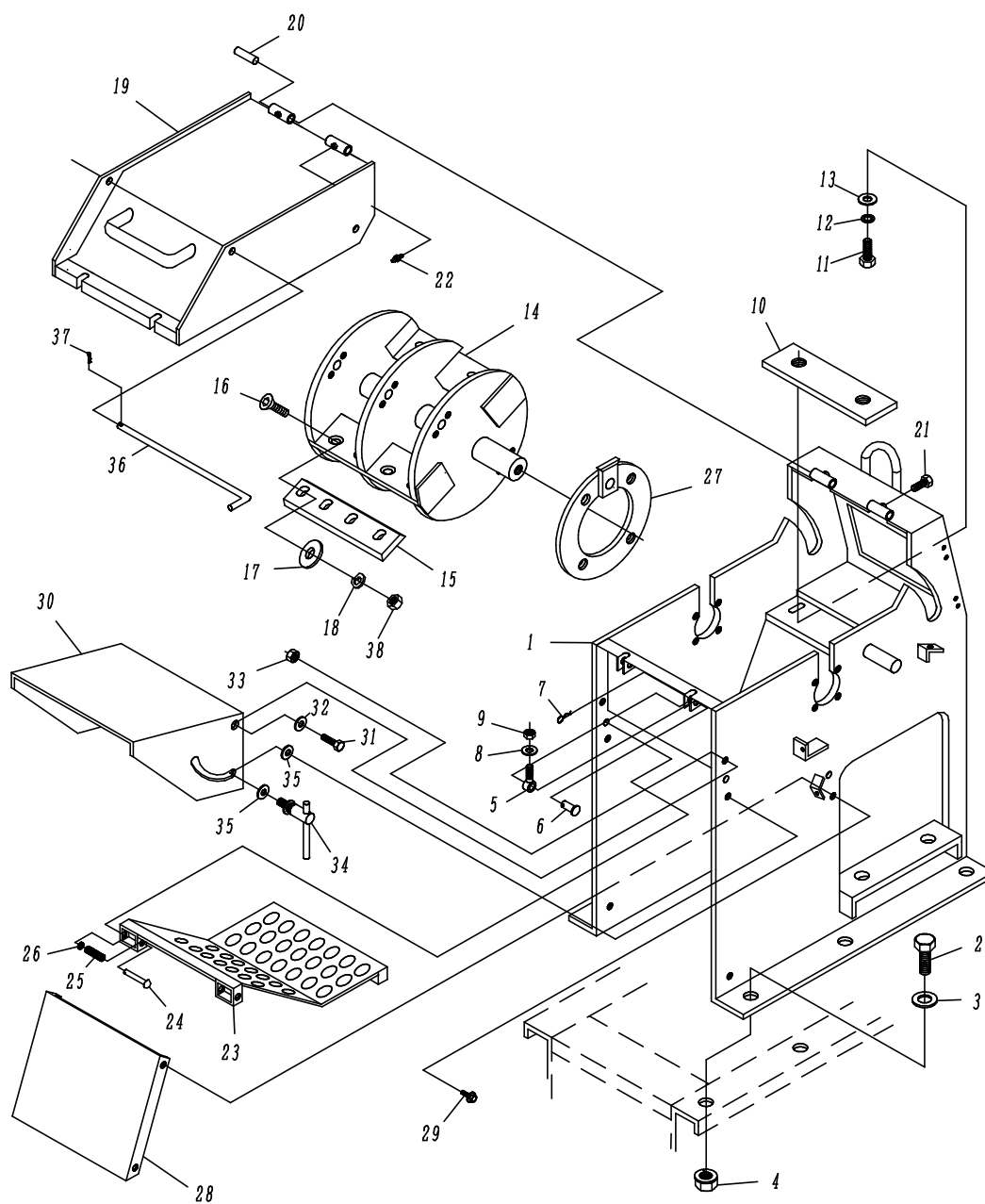
Fig. 6 ロータ系
