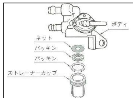
燃料コック
