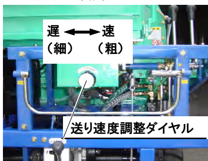
送り速度調整ダイヤル
