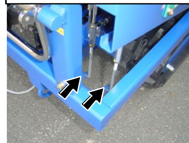
サイドクラッチリンク
