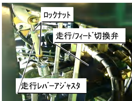
走行レバーアジャスタ
