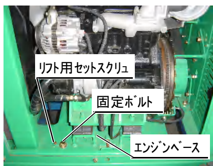
エンジンベース
