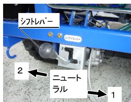
シフトレバー
