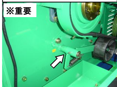
テンションアーム
