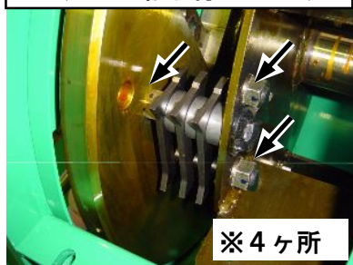
シュレッダーナイフ軸取付ボルト・ナット
