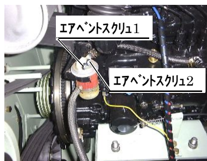
燃料フィルタ
