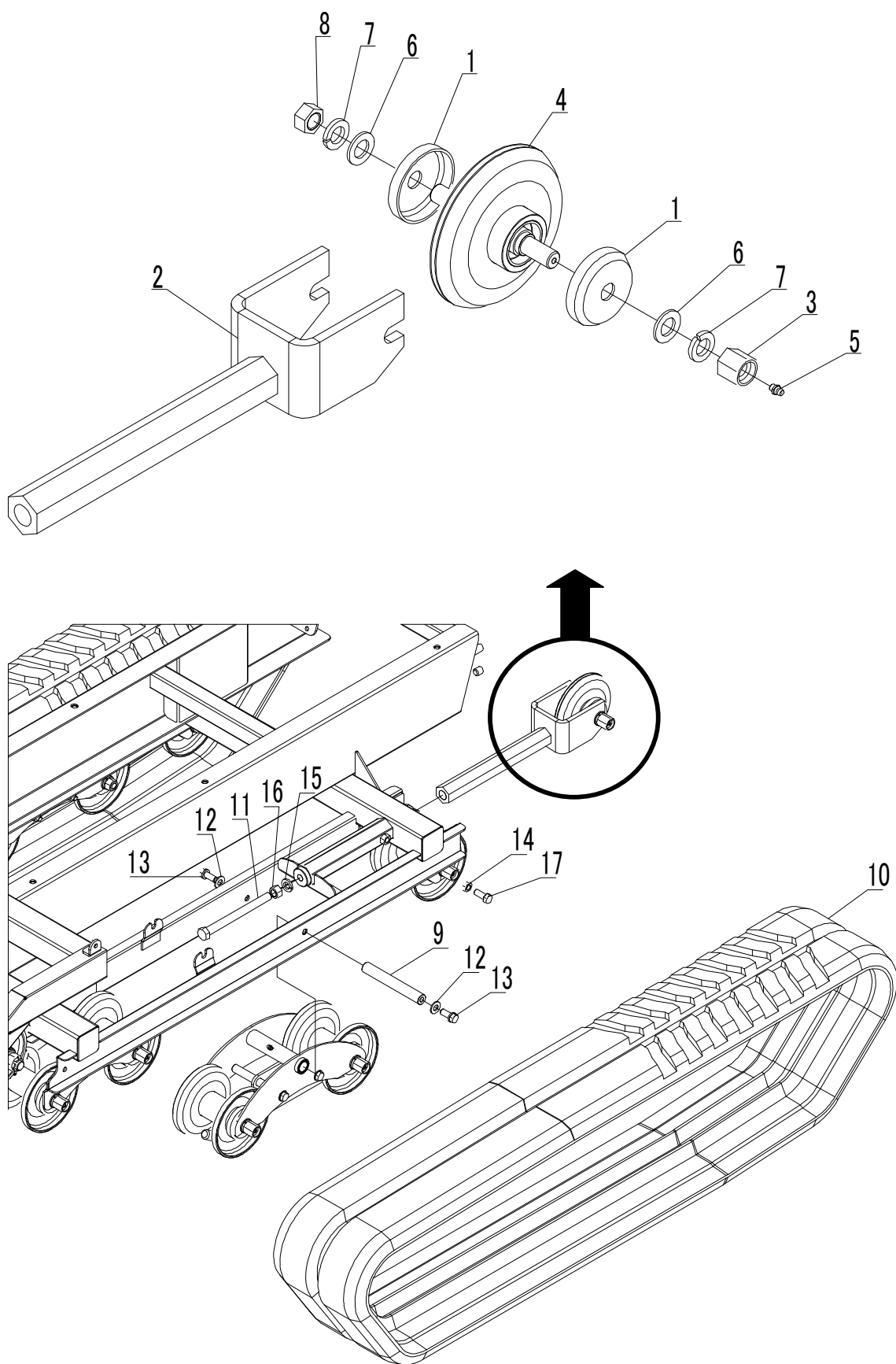
Fig. 3 誘導輪系
