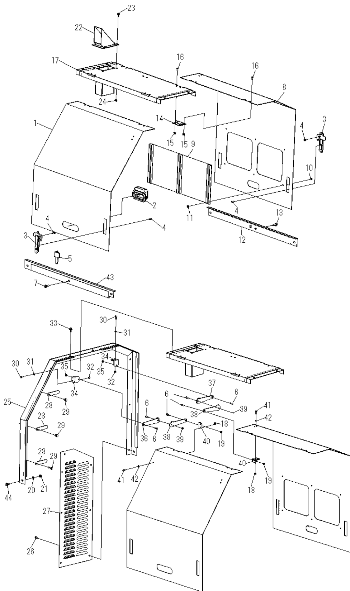
Fig. 17-2 カバー系
