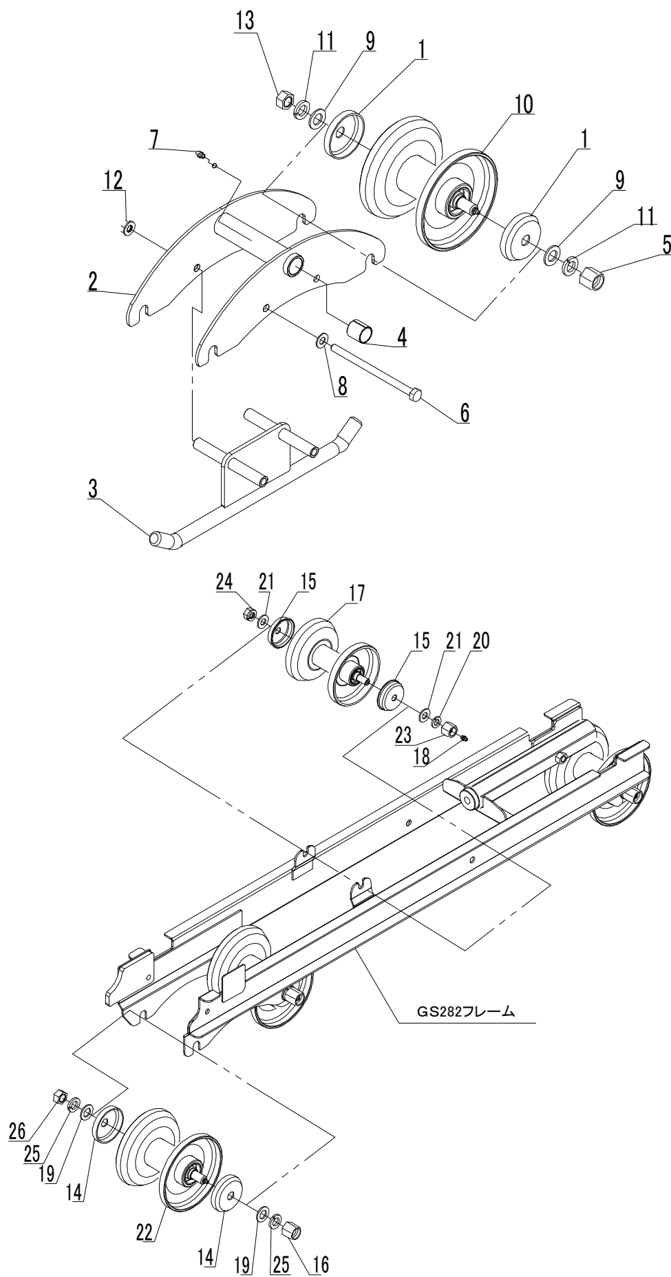
Fig. 2 転輪系
