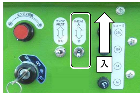
ロータクラッチスイッチ
