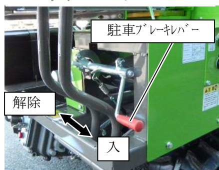
駐車ブレーキレバー
