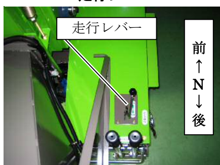
走行レバー
