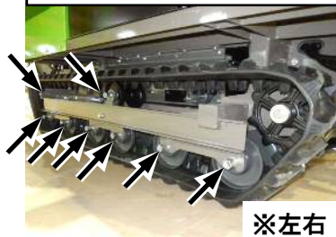
転輪・誘導輪固定ナット
