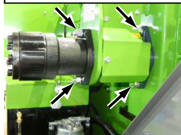
送りモータ・軸受取付部
