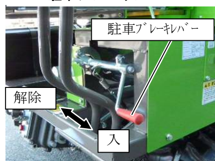
駐車ブレーキレバー
