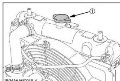
①ラジエータキャップ
