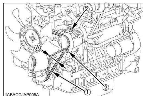
①ファンベルト ②ボルト、ナット
