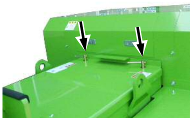
ロータバー固定ナット
