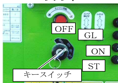
エンジンキー
