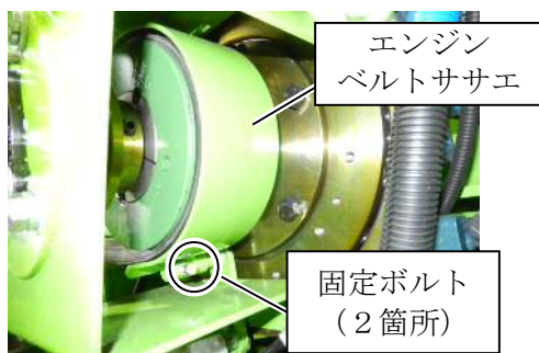
エンジンベルトササエ
