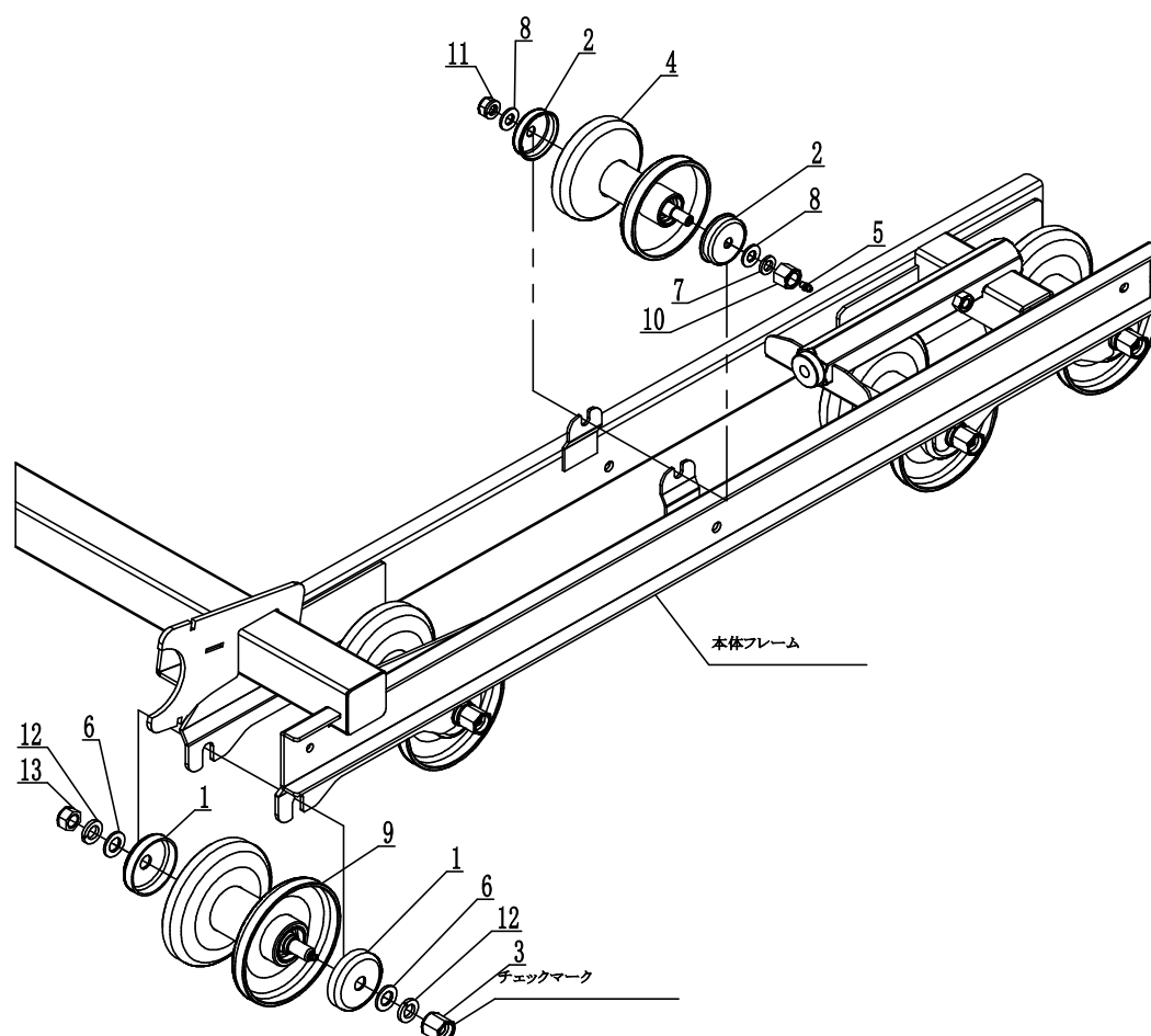
Fig. 5 転輪取付
