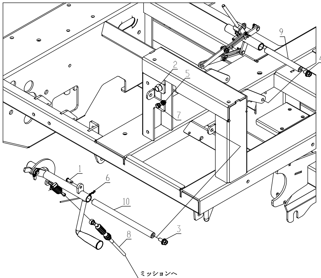
Fig. 11 駐車ブレーキワイヤー取付(1)
