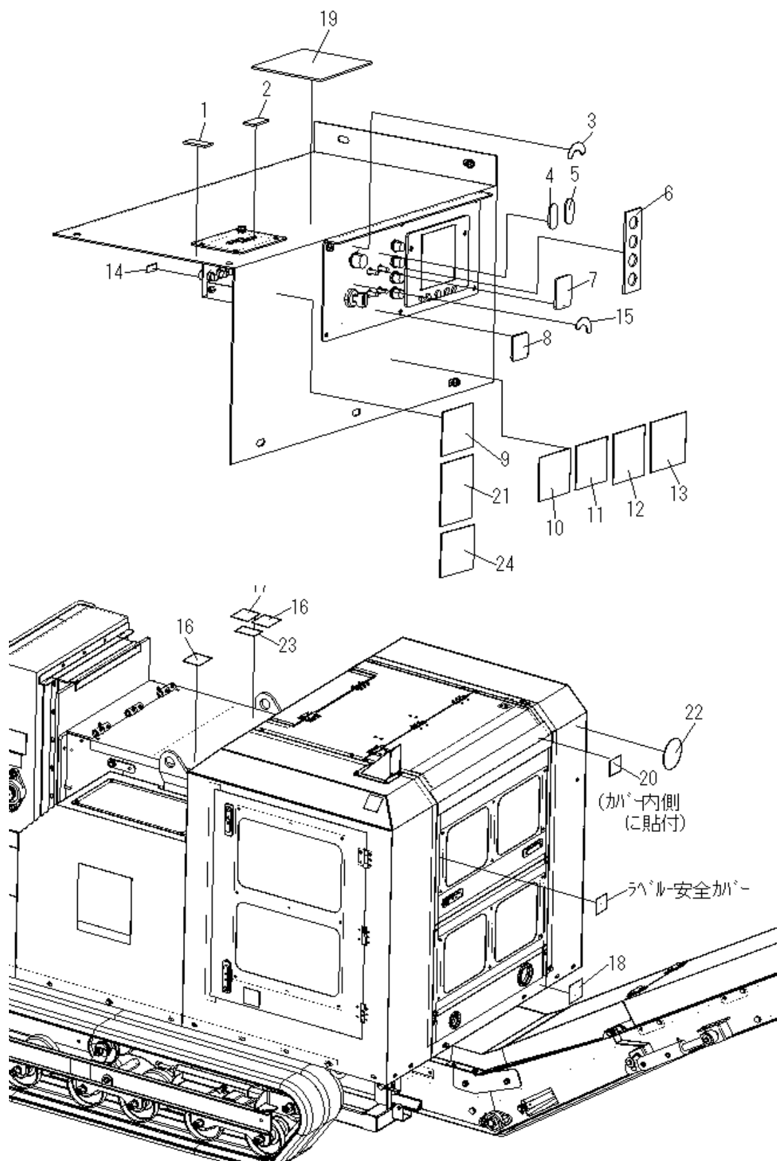
Fig. 25-2 ステッカー
