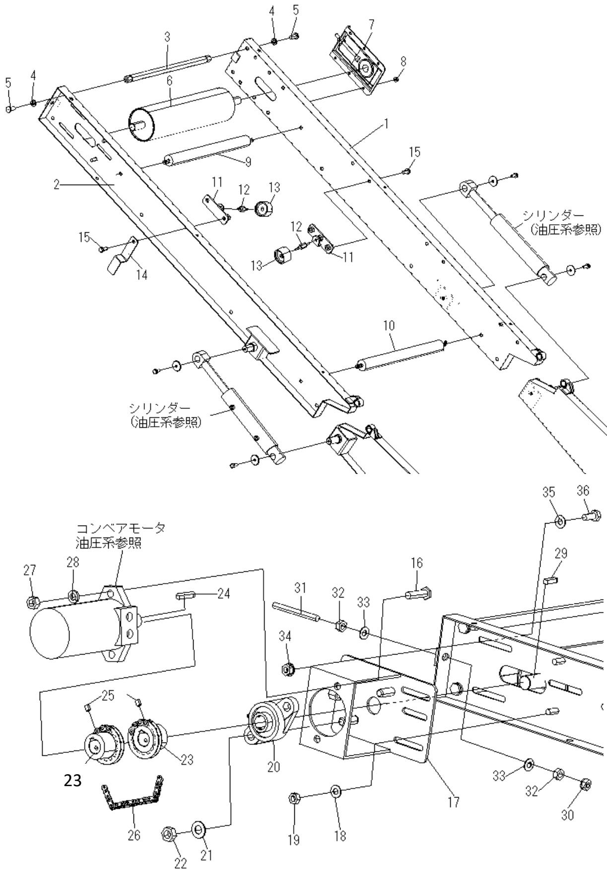
Fig. 23-2 排出コンベア
