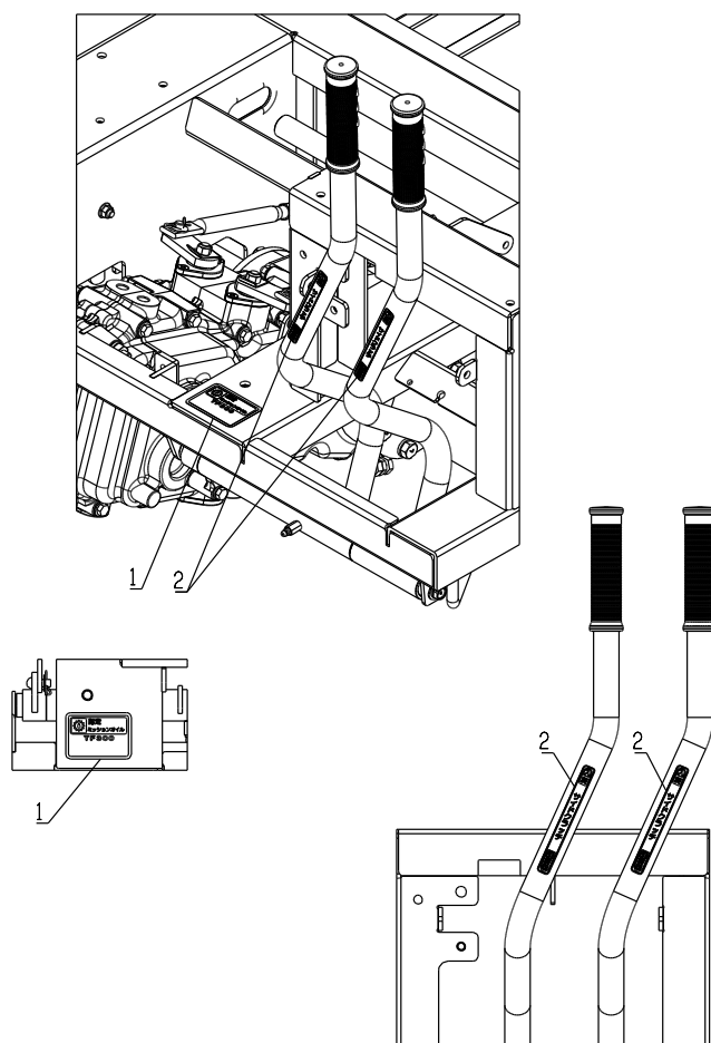
Fig. 14 ステッカー
