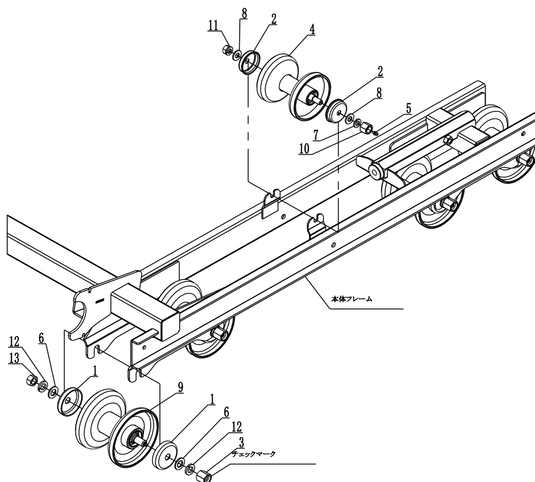
Fig. 5 転輪取付
