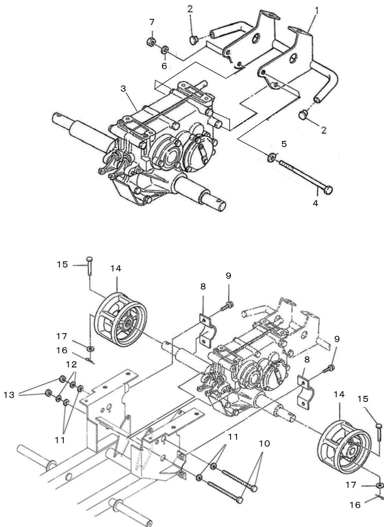
Fig.1 フレーム系(1)
