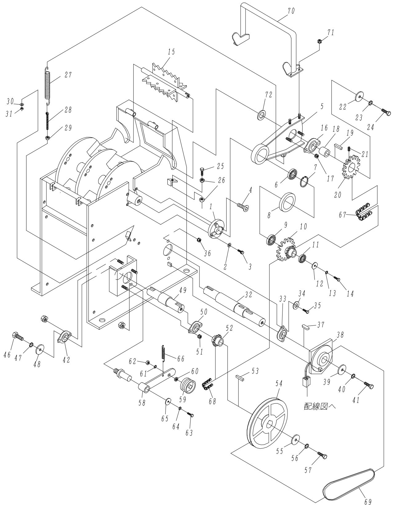
Fig.9 ローターハウジングL
