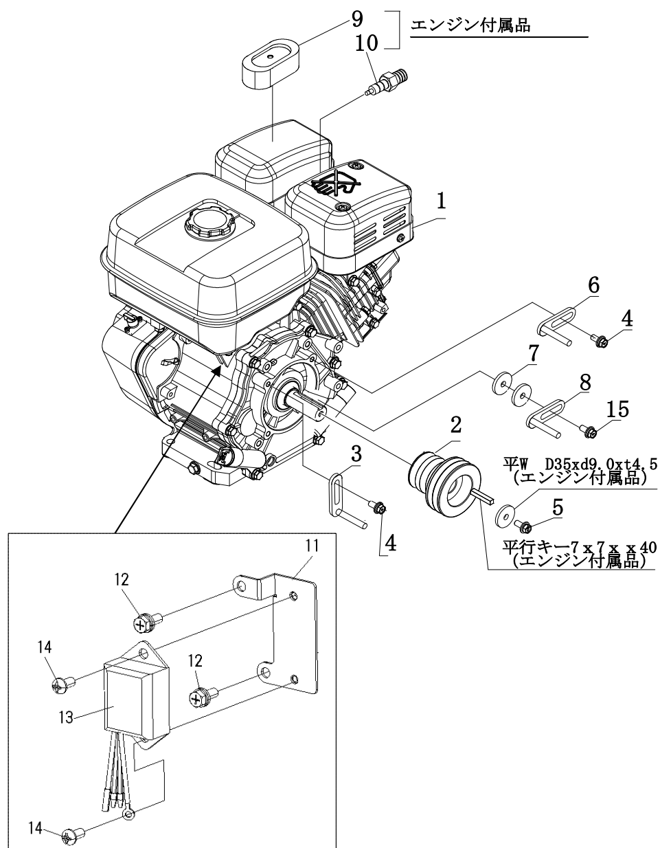
Fig. 6 エンジン系①
