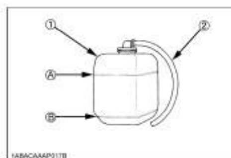
①リザーブタンク ②オーバフローパイプ A“上限” [FULL] B“下限” [LOW]
