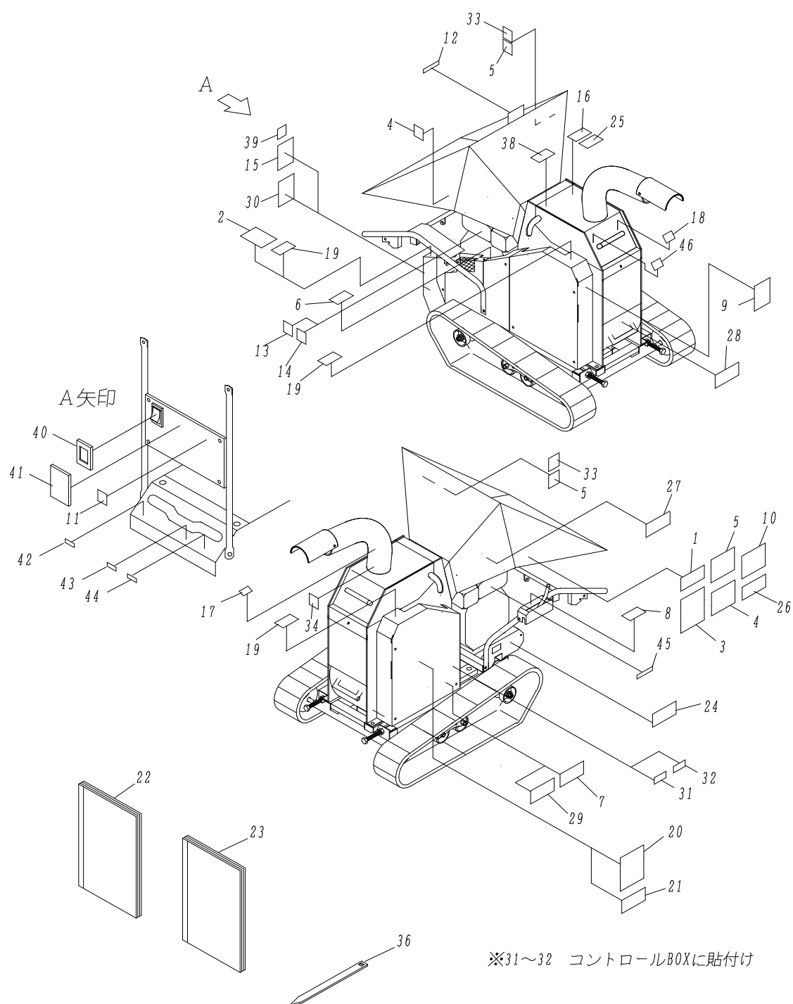
Fig.12 ステッカー・付属品(2)
