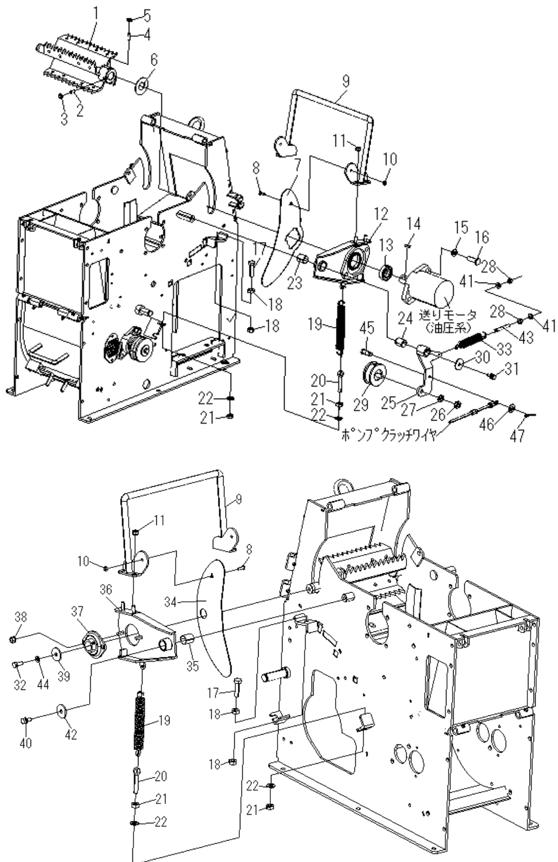
Fig. 11 フィーダ系
