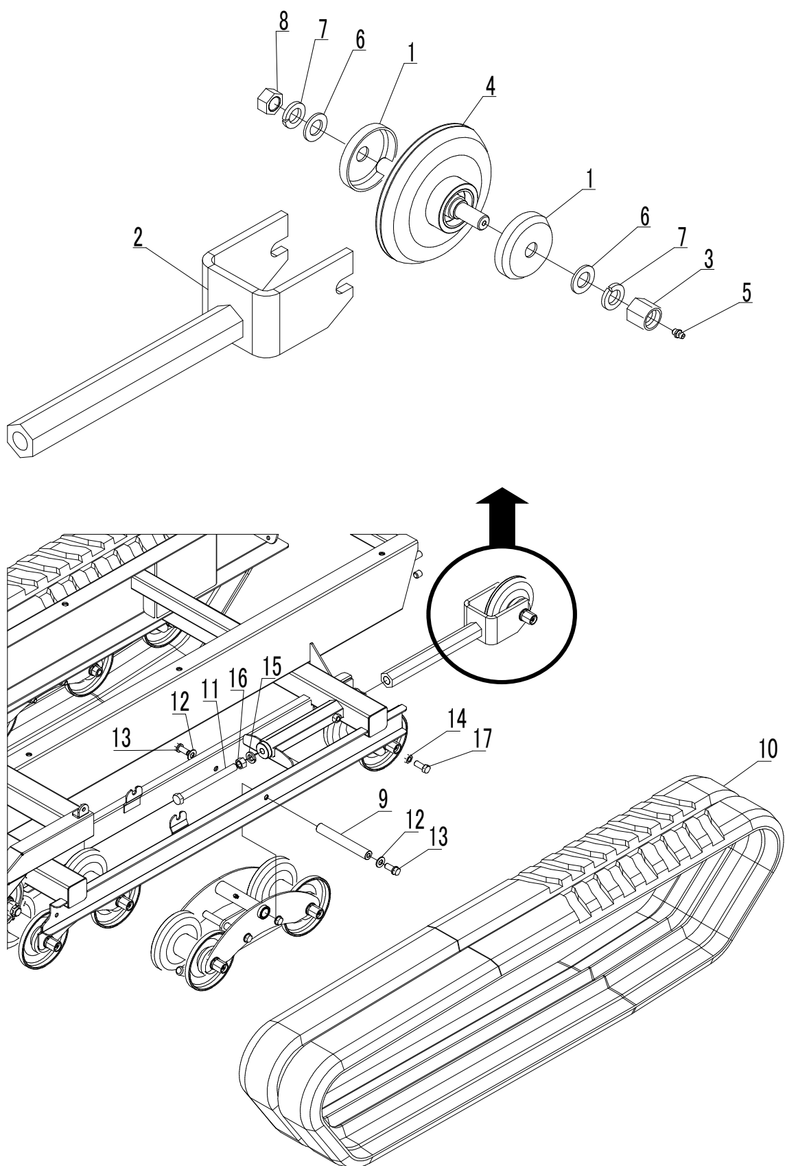
Fig. 3 誘導輪系
