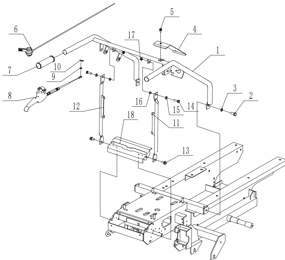
Fig. 4 ハンドル
