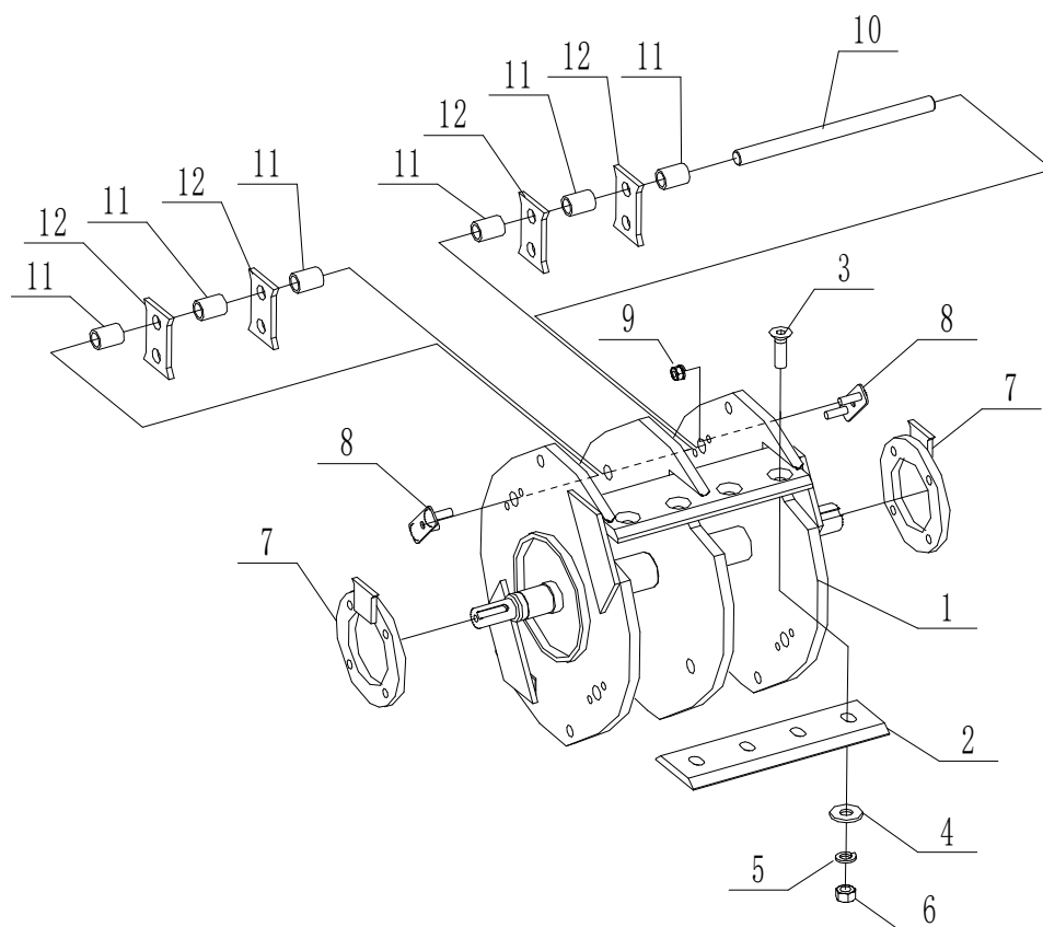
Fig. 14 ロータジク
