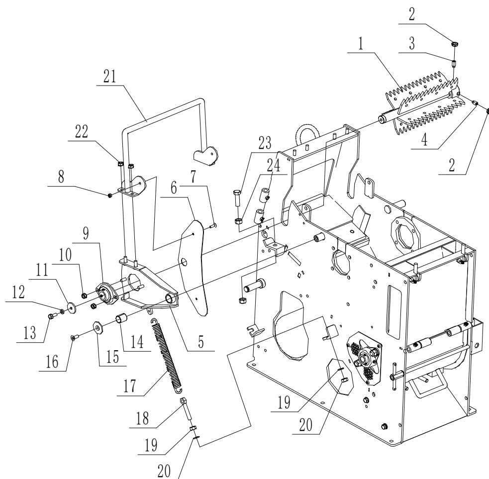
Fig. 24 フィードアームR
