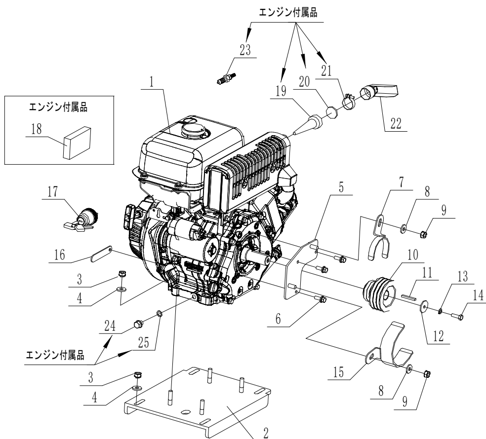
Fig. 12 エンジン
