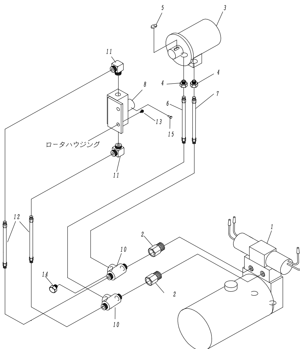
Fig. 10 油圧系
