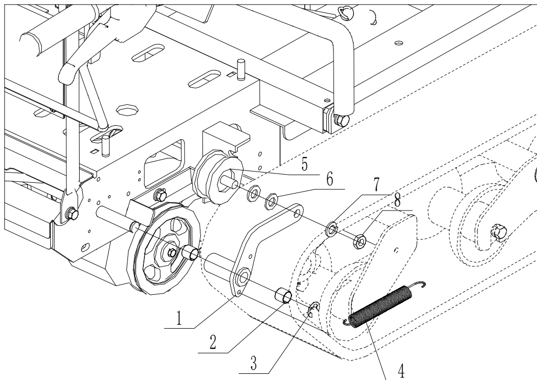
Fig. 8 Mテンションアーム
