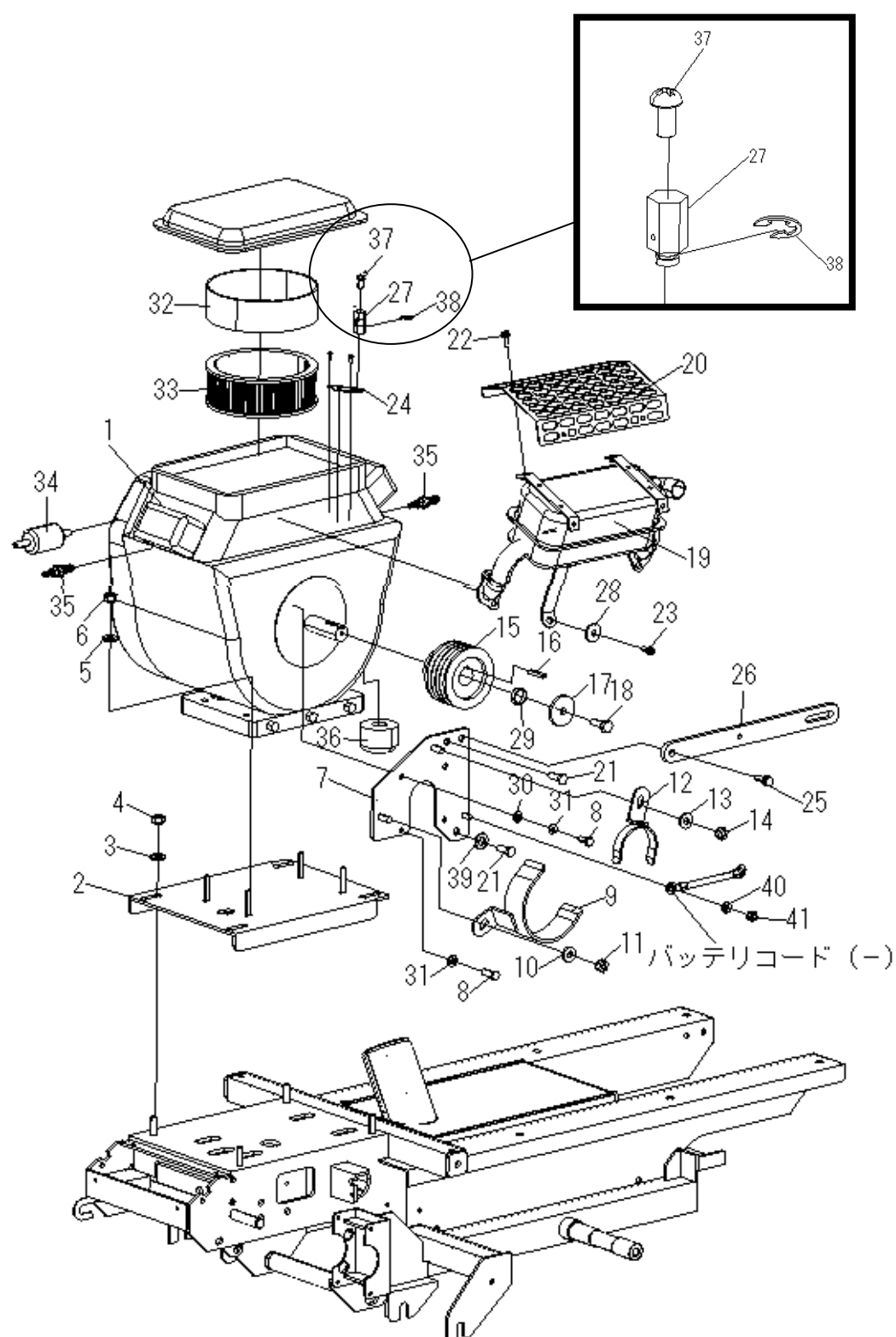
Fig. 4 エンジン系
