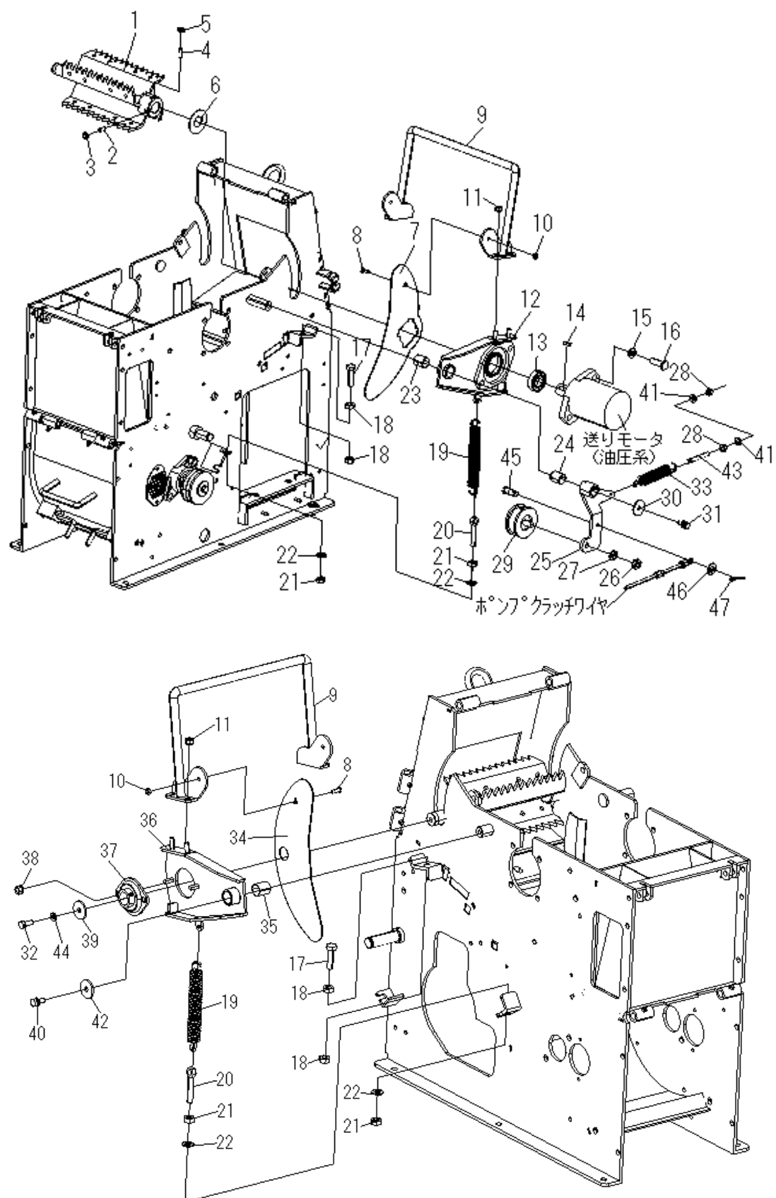
Fig. 11 フィーダ系
