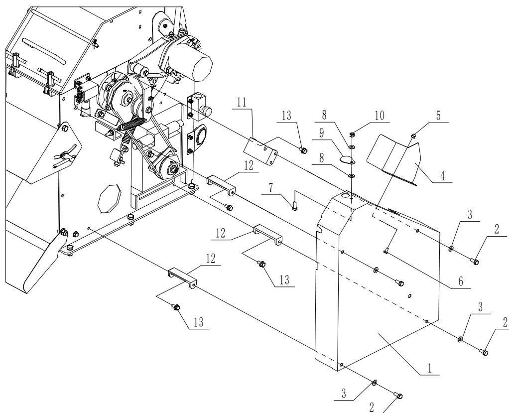
Fig. 26 カバーL
