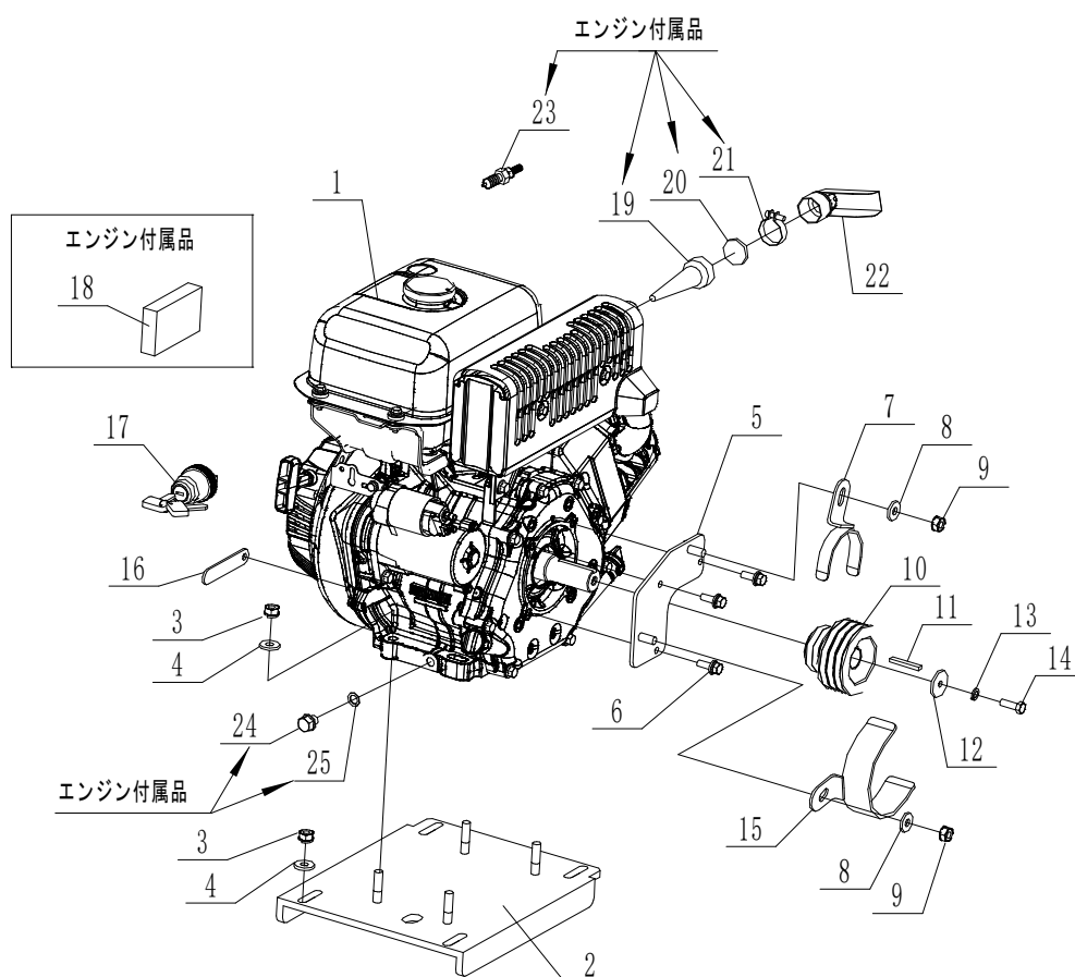
Fig. 12 エンジン
