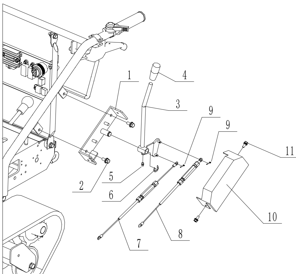
Fig. 7 Rレバー
