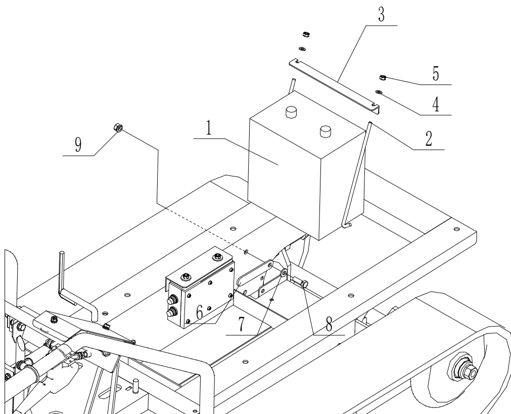
Fig. 9 バッテリ
