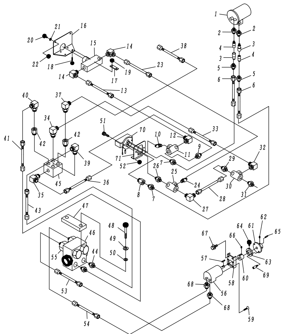
Fig. 3-1 油压系 (2)
