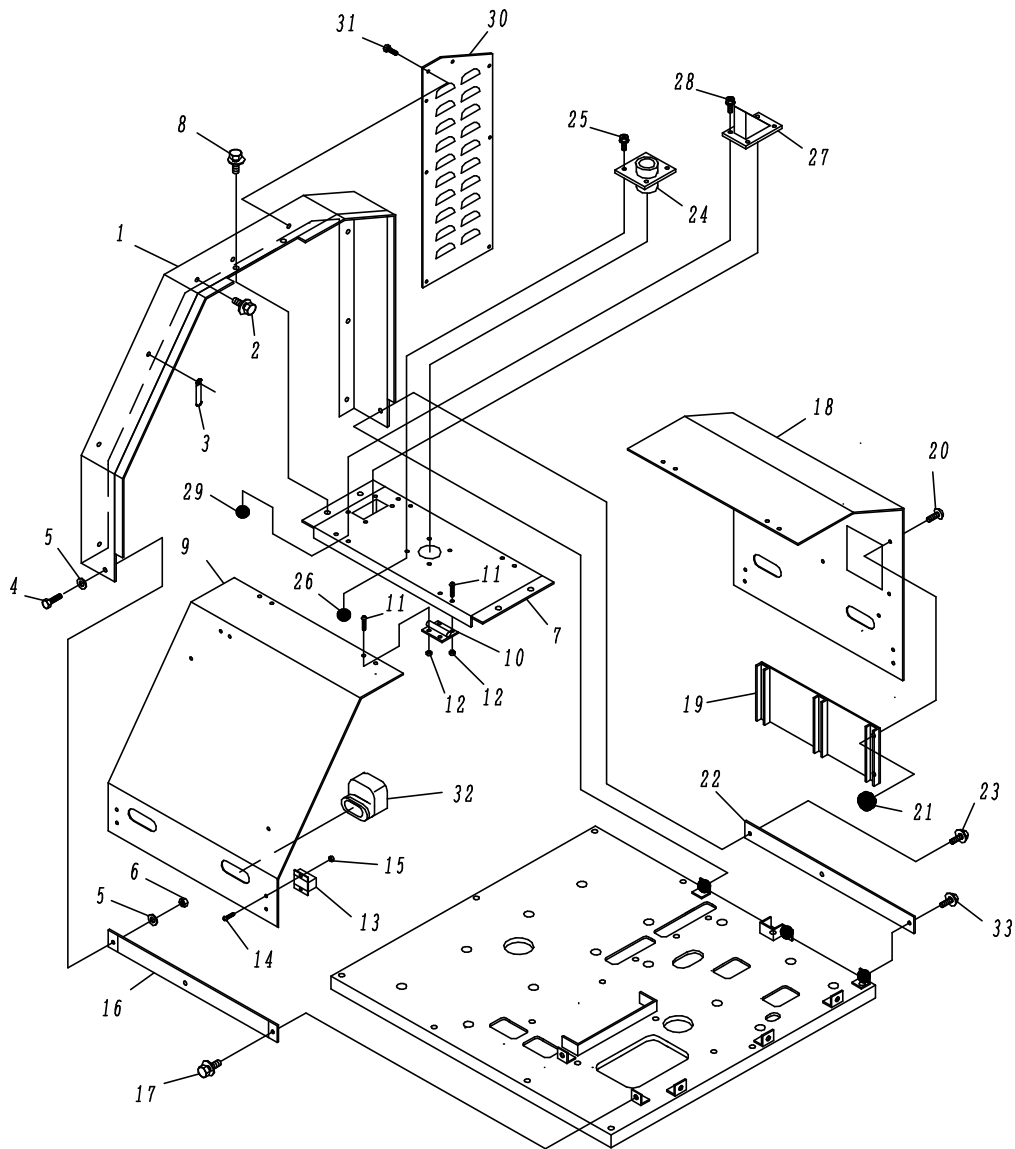
Fig. 9-1 カバー系
