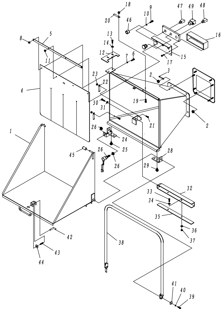
Fig. 8 ホツパ系
