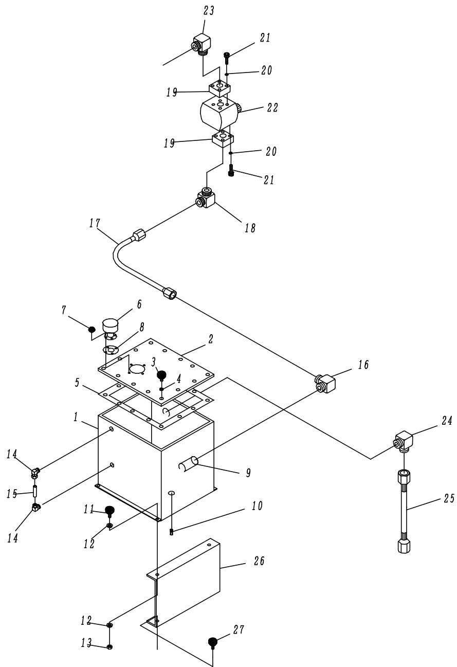
Fig. 3-2 油压系
