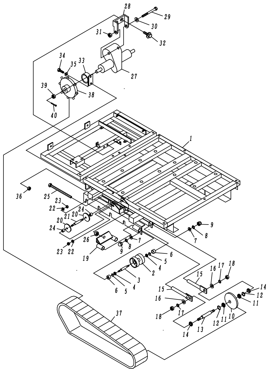
Fig. 1-1 フレーム系
