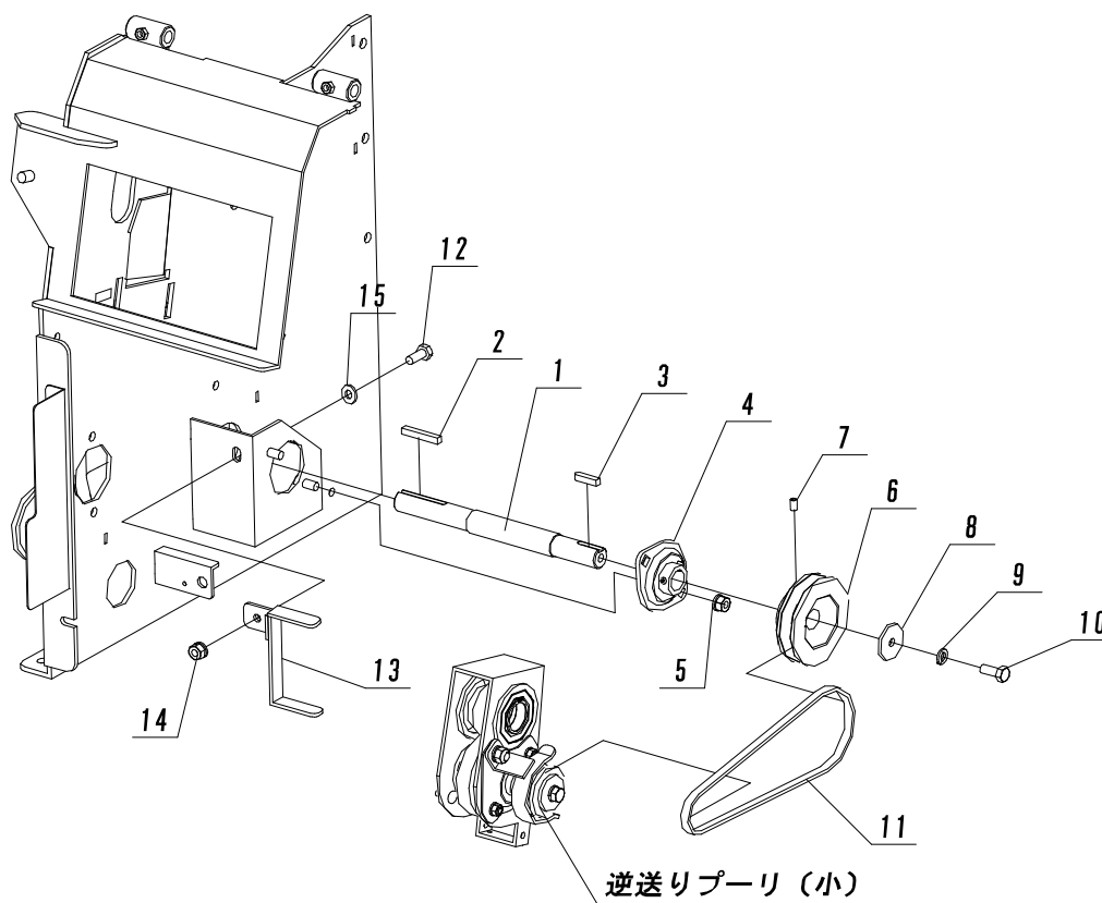
Fig. 17 ロータハウジング⑧(第二中間軸①)
