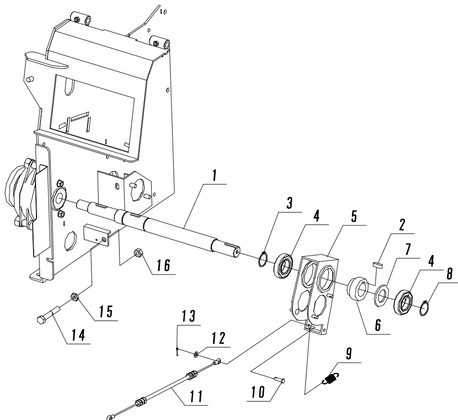
Fig. 14 ロータハウジング⑤(第一中間軸①)
