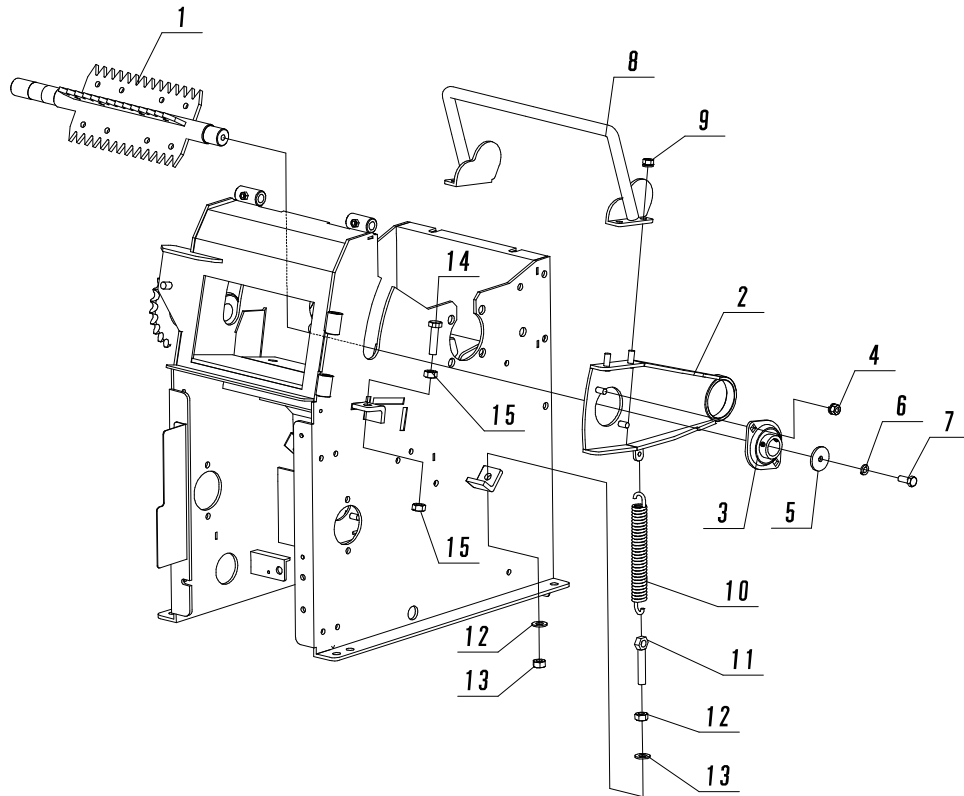
Fig. 20 フィードローラ①
