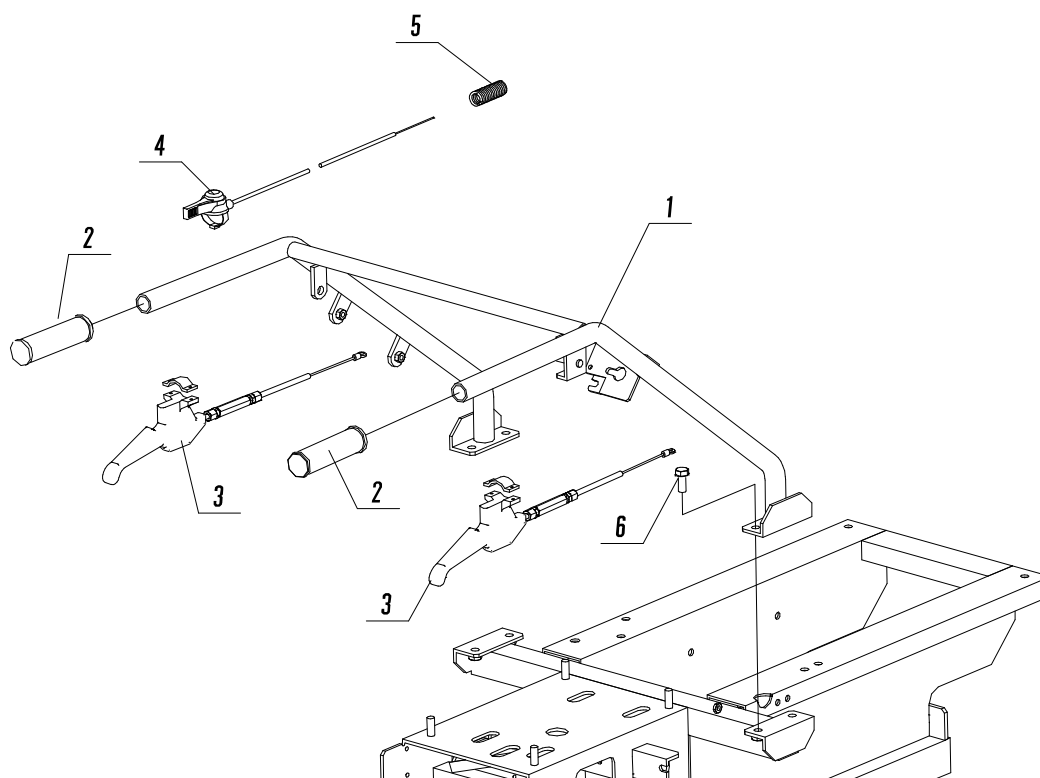
Fig. 5 ハンドル
