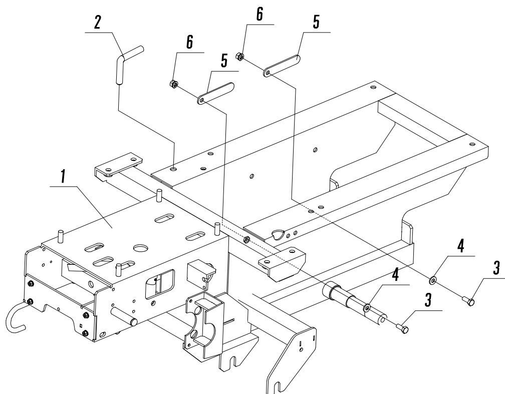
Fig. 1 メインフレーム
