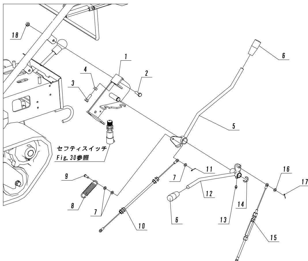
Fig. 7 Rレバー
