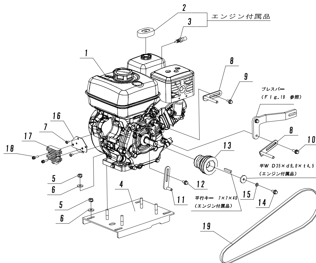
Fig. 9 エンジン
