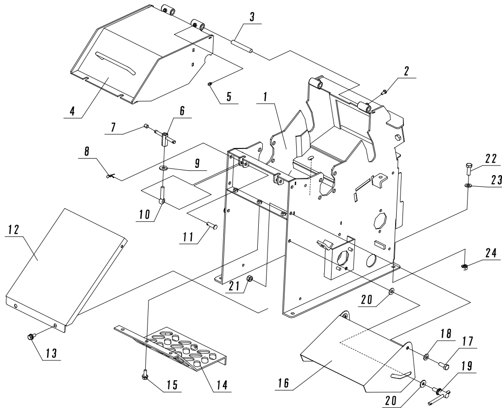
Fig. 10 ロータハウジング①
