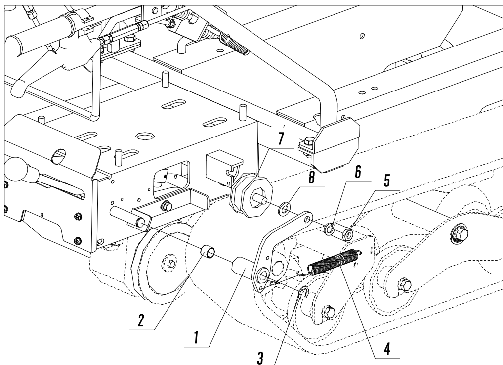
Fig. 8 Mテンションアーム
