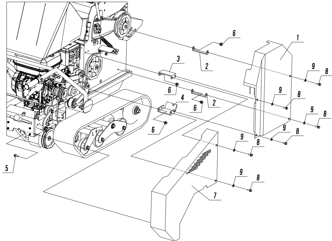
Fig. 23 カバー-R
