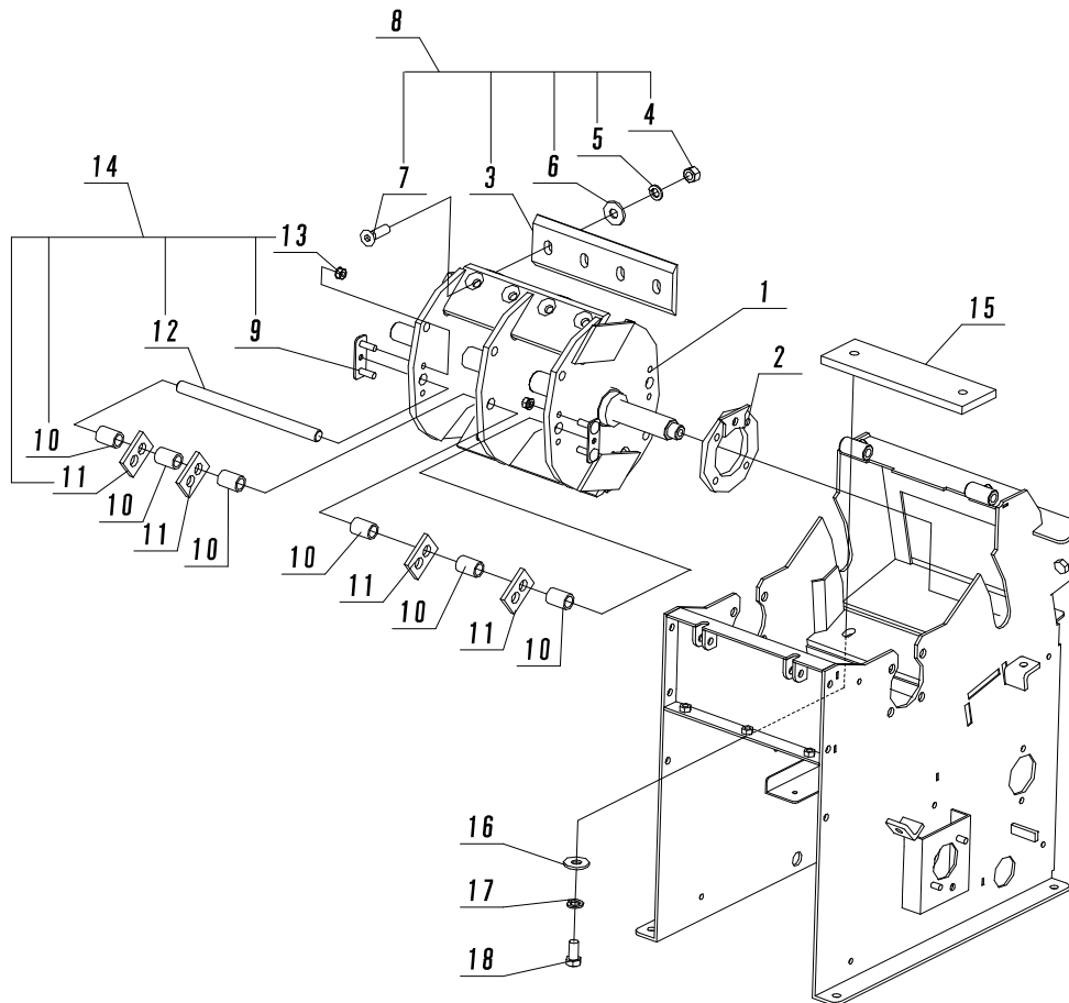
Fig. 11 ロータハウジング②
