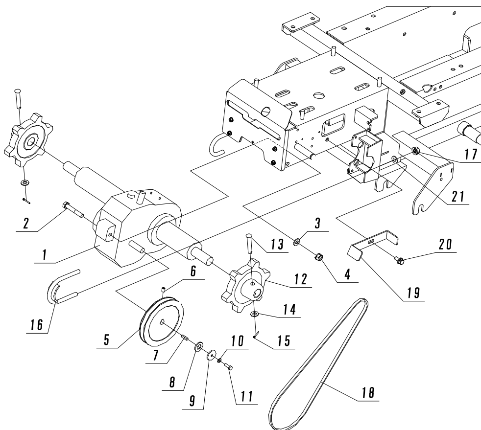
Fig. 3 走行ミッション
