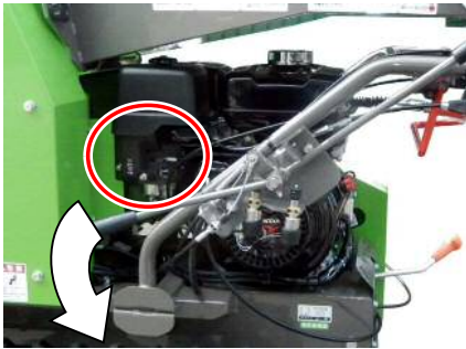
燃料コック
