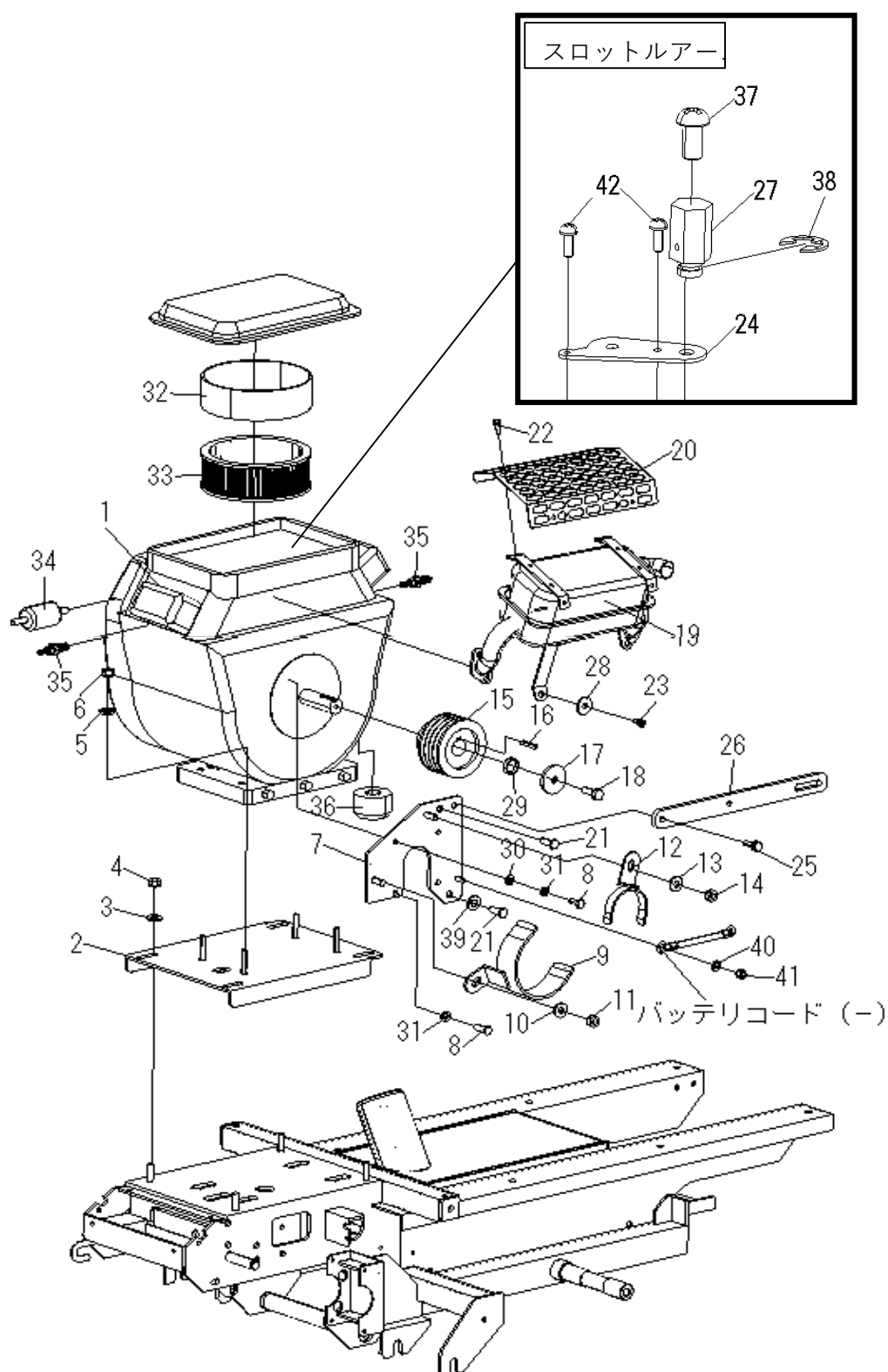
Fig. 4 エンジン系
